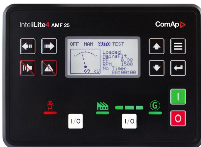
Obr. 4.2 Produkt AMF25
