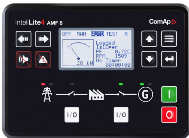
Obr. 4.1 Produkt AMF8
