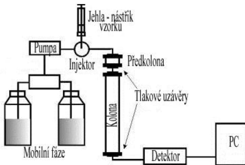
Obrázek 7 - Schéma HPLC [49]
