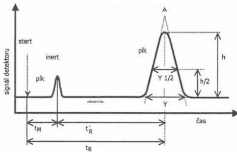
Obrázek 8 - Ukázka chromatogramu [52]
