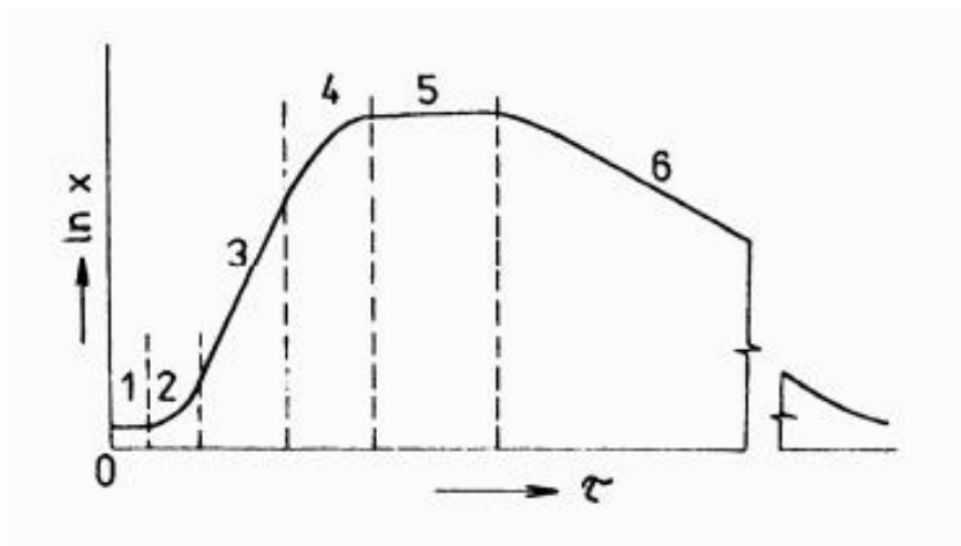
Obrázek 5 - Růstová křivka [35]
