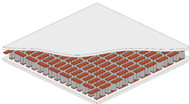
Obr. 2 Termoelektrický modul
