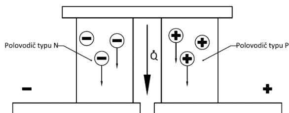
Obr. 1 Termoelektrická dvojice
