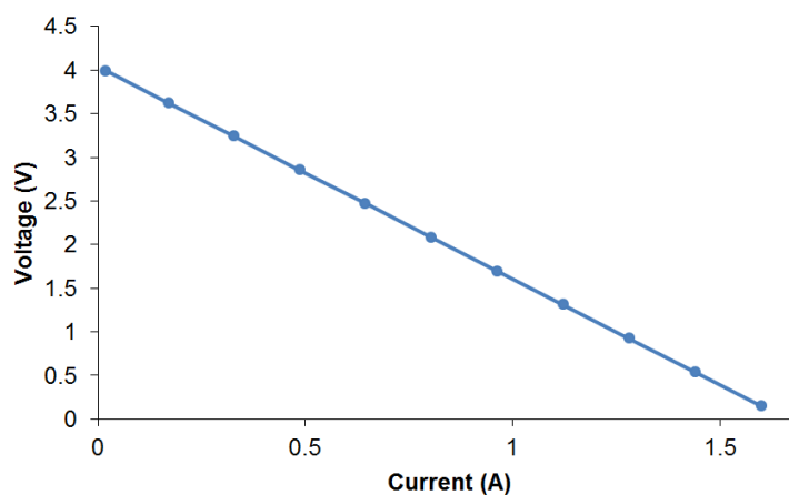
Obr. 9 Zatěžovací charakteristika BiTe modulu při t_h=170\text{ }^\circ\text{C} a t_c=70\text{ }^\circ\text{C} [17]
