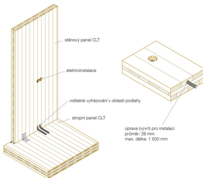
Obrázek 13 Vedení elektroinstalace
