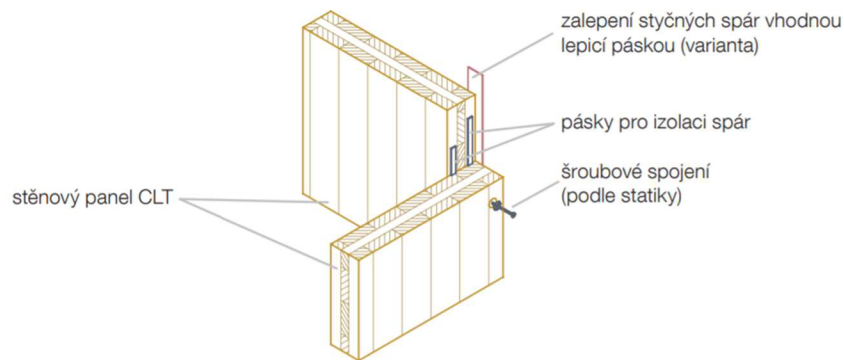
Obrázek 8 Rohový spoj
