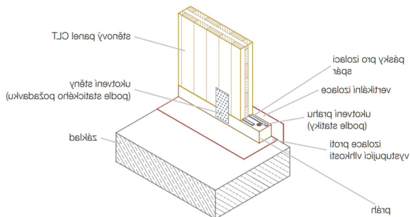
Obrázek 7 Založení soklu
