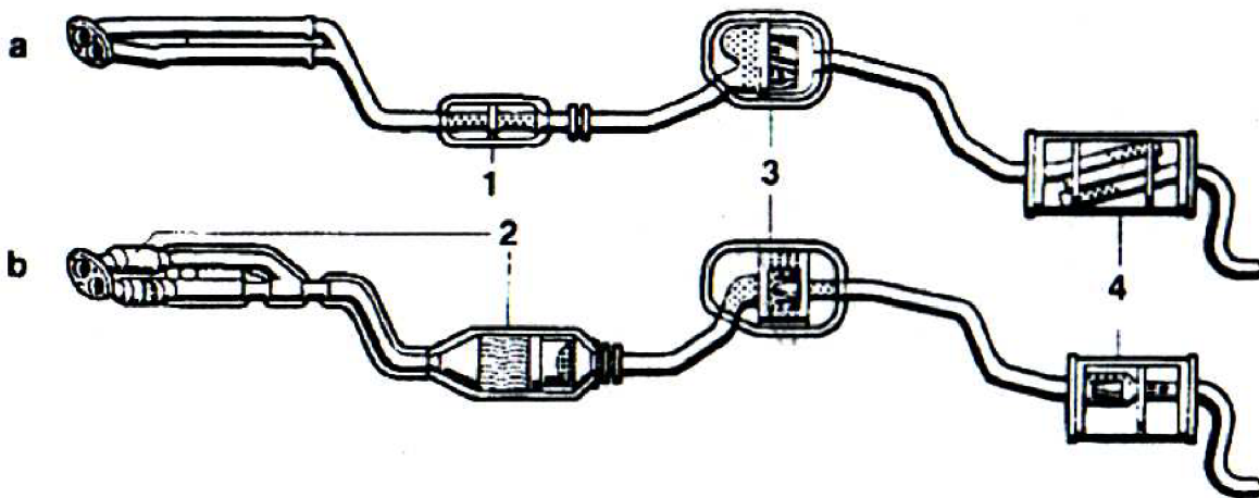
Obr. 2.2 Výfukové systémy: [2] a – bez katalyzátoru, b – s katalyzátorem 1- přední tlumič hluku, 2- katalyzátor, 3 – střední tlumič hluku, 4 – koncový tlumič hluku
