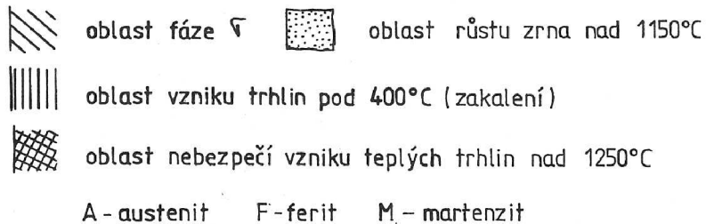
Obr. 5.4 Oblast fázového složení základního materiálů označena zeleně [11]
