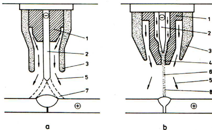
Obr. 4.4 Princip svaření [9]
