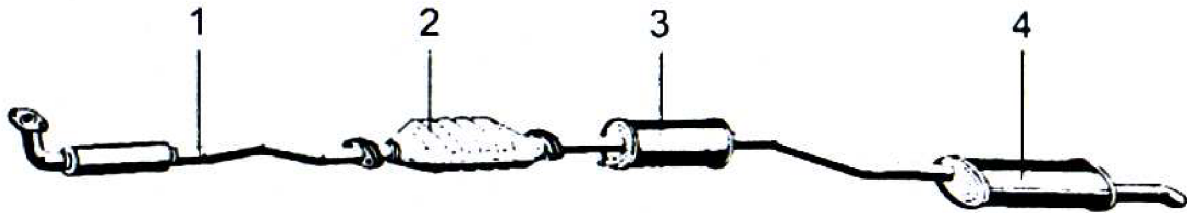
obr. 2.1 Výfukový systém pro osobní automobil (výfukové sběrné potrubí nezakreslené ): [2] 1- přední výfukové potrubí, 2- katalyzátor, 3- předřazený (střední) tlumič hluku, 4- zadní (koncový) tlumič hluku s koncovým potrubím
