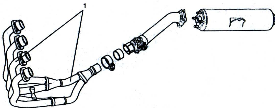
Obr. 2.10 Jedno trubkový výfuk čtyřválcového čtyřdobého motoru se čtyřmi koleny a s tlumičem (Suzuki GSX-R 1000). [3]
