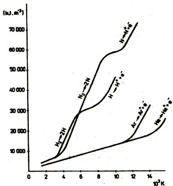
Obr. 4.1 Závislost entalpie plynů na teplotě [9]
