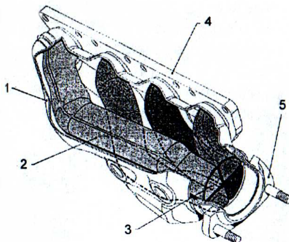
Obr. 2.4 Plechové výfukové sběrné potrubí izolované vzduchovou mezerou (zážehový motor Audi V8, MTZ 1991/1): [2] 1 – plechový kryt, 2 – samostatné výfukové trubky tvářené vysokým vnitřním tlakem, 3 – čtyři sběrná výfuková potrubí, 4 – příruba výfukového sběrného potrubí (levá řada válců), 5 – připojení k přednímu potrubí výfukového systému (příruba sběrného výfukového potrubí)
