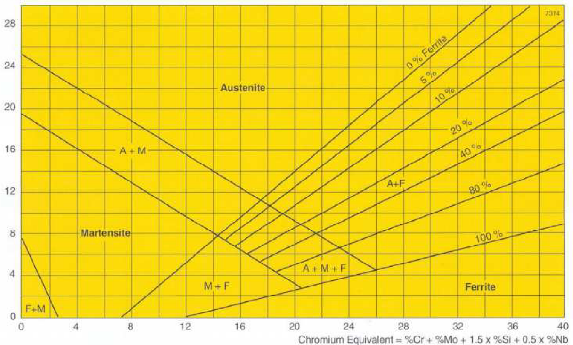
Obr. 3.7 Schaefferův diagram znázorňující strukturu svarového kovu korozi vzdorných ocelí podle účinného obsahu chrómu a niklu [10]
