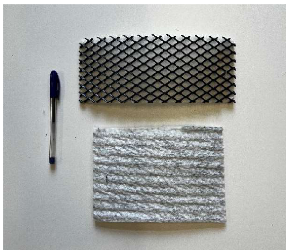
Obrázek 44: Geokompozit (Nývtl, 2023)
