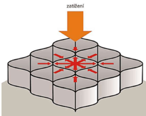
Obrázek 41: Rozklad zátížení v geobuňce (Vysoká škola báňská – Technická univerzita Ostrava, © 2012)
