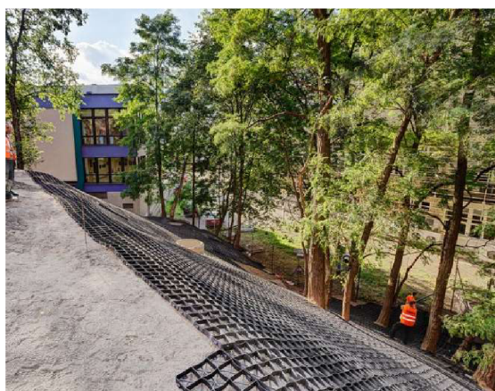
Obrázek 38: Instalace plastové zatravnovací dlaždice (PROSTAVBU, © 2022)
