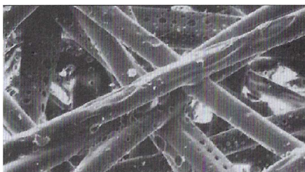
Obrázek 2: Tepelně pojená geotextilie netkaná (Ponikelský a kol., 2011)
