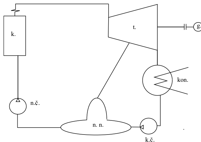
Obr. 3 Rankin-Clausiusův oběh
