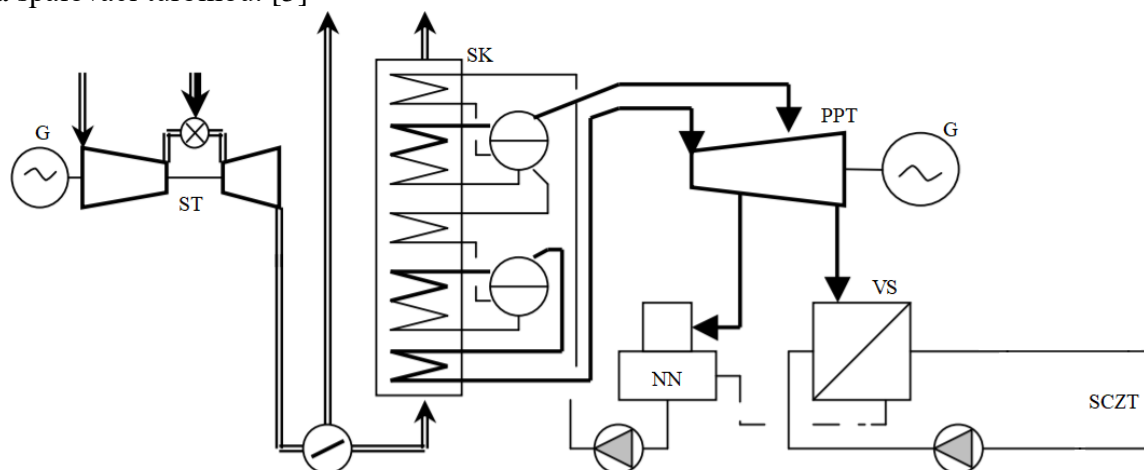
Obr. 10 Základní schéma zapojení zdroje v paroplynovém cyklu [5]
