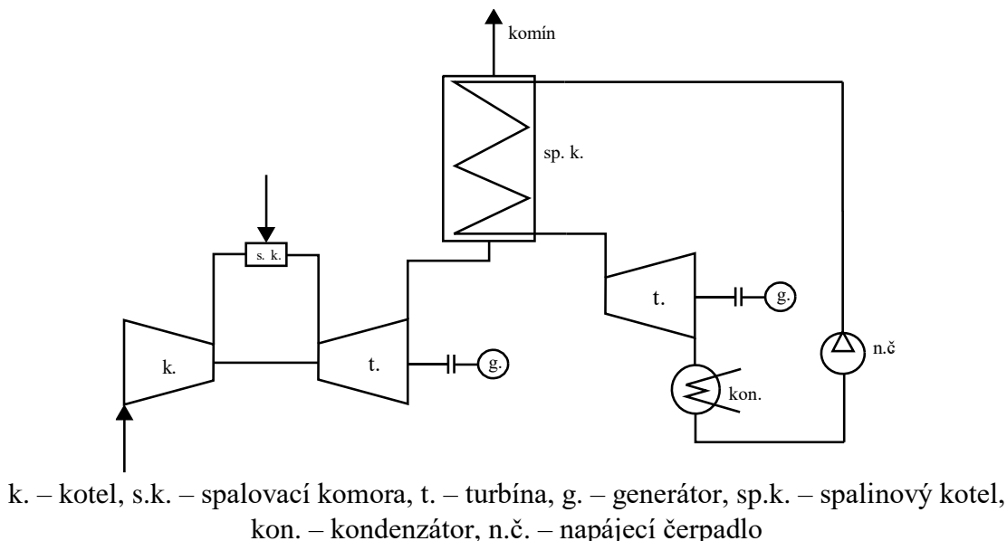
Obr. 5 Paroplynový oběh
