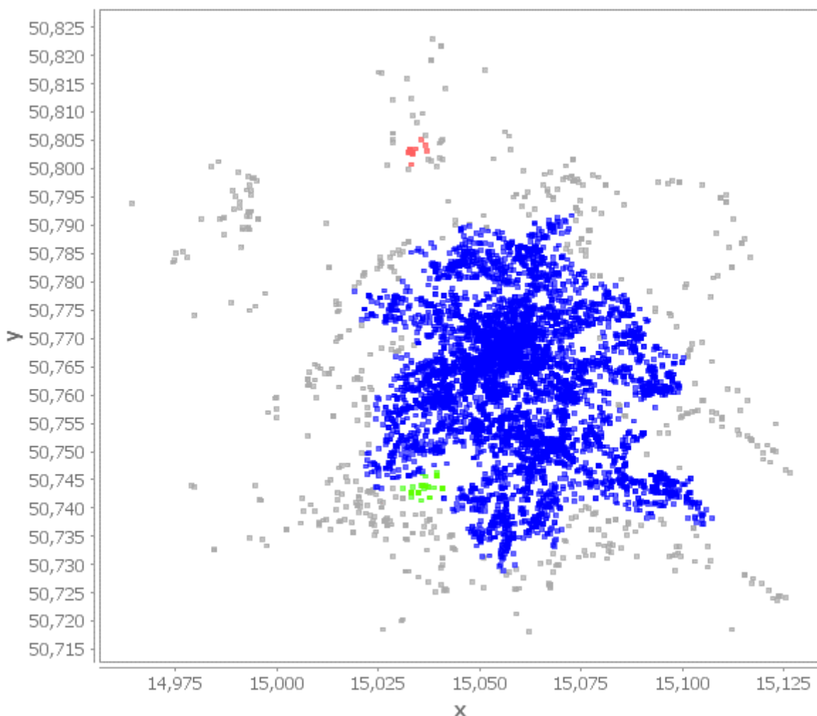
Obr. 33 – Přehled shluků DBSCAN pro MinPts = 20, Vzdálenost 200 m
