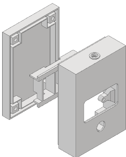
Obrázek 8 Model krabičky
