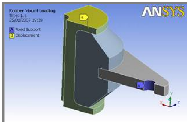
Obr. 9 Okrajové podmínky aplikovány na geometrických Entitách [3]
