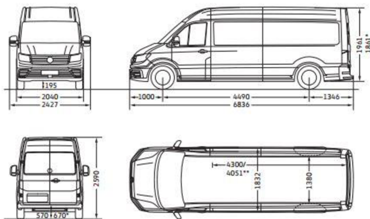
Crafter 35 skříňový vůz dlouhý rozvor s vysokou střechou
