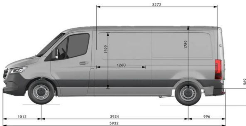
Obrázek 8 Rozměry Mercedes-Benz střední délky
