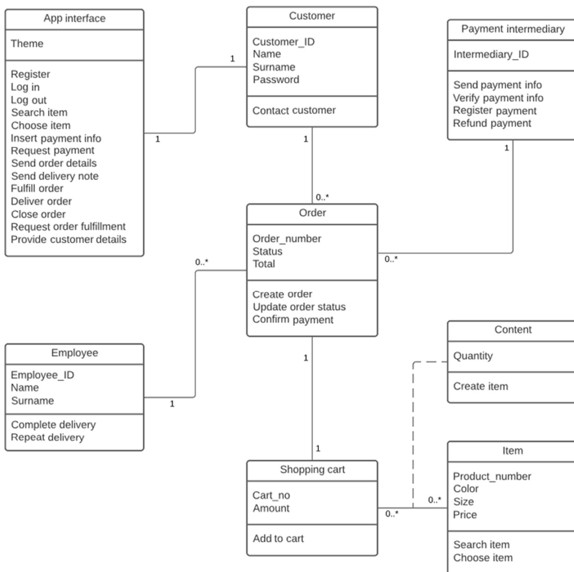
Obrázek 19 - Diagram tříd
