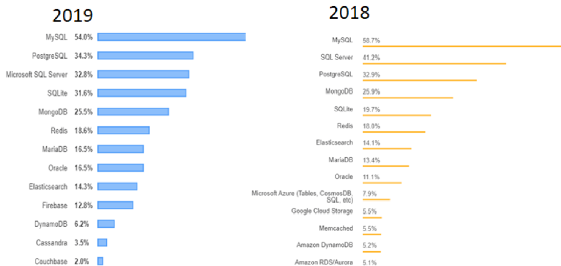
Obrázek 12 - Nejoblíbenější DMBS 2019, 2018 Zdroj – [20][21]
