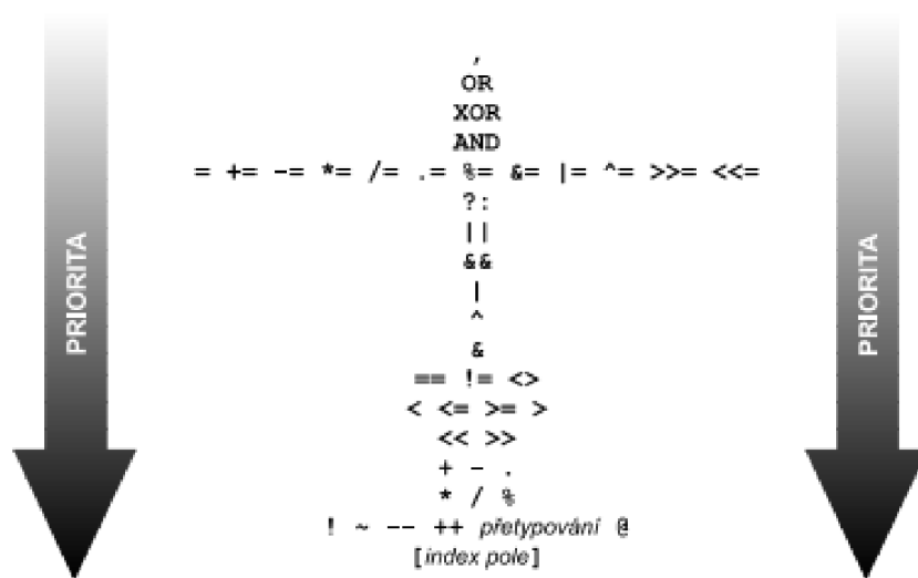
Obrázek 7 - priorita PHP operátorů Zdroj - [10]
