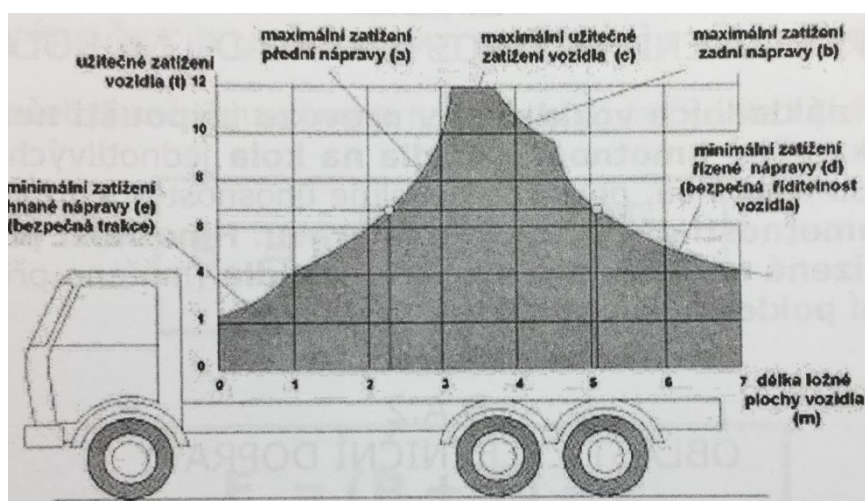
Obr. 1.26 Graf zatížitelnosti/rozložení nákladu
