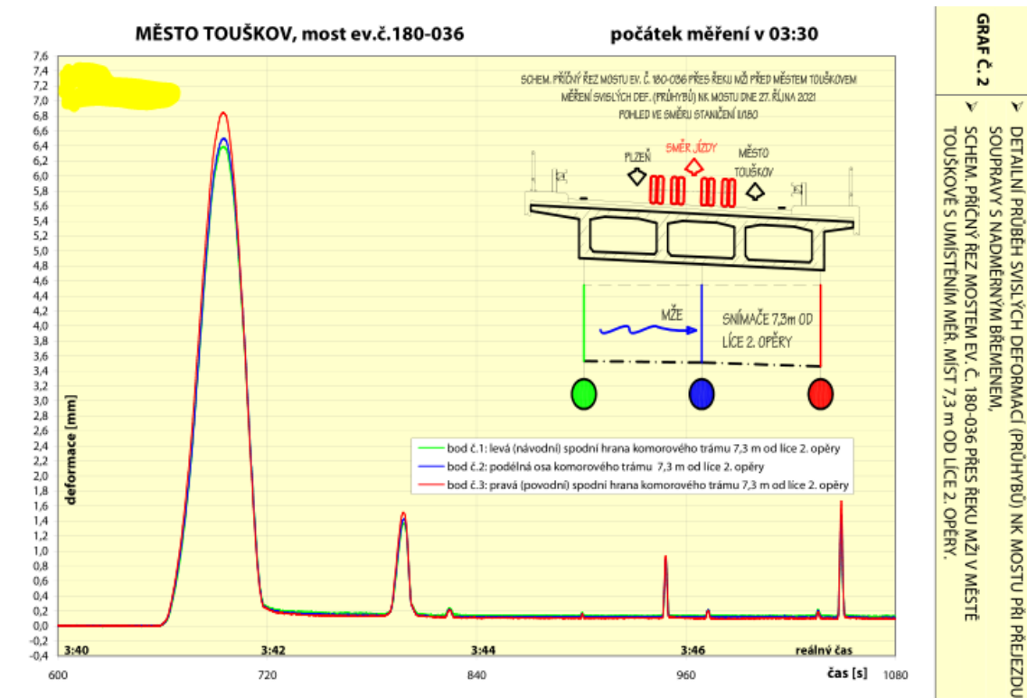
Obr. 4.14 Záznam ze sledování svislých deformací nosné konstrukce mostu
