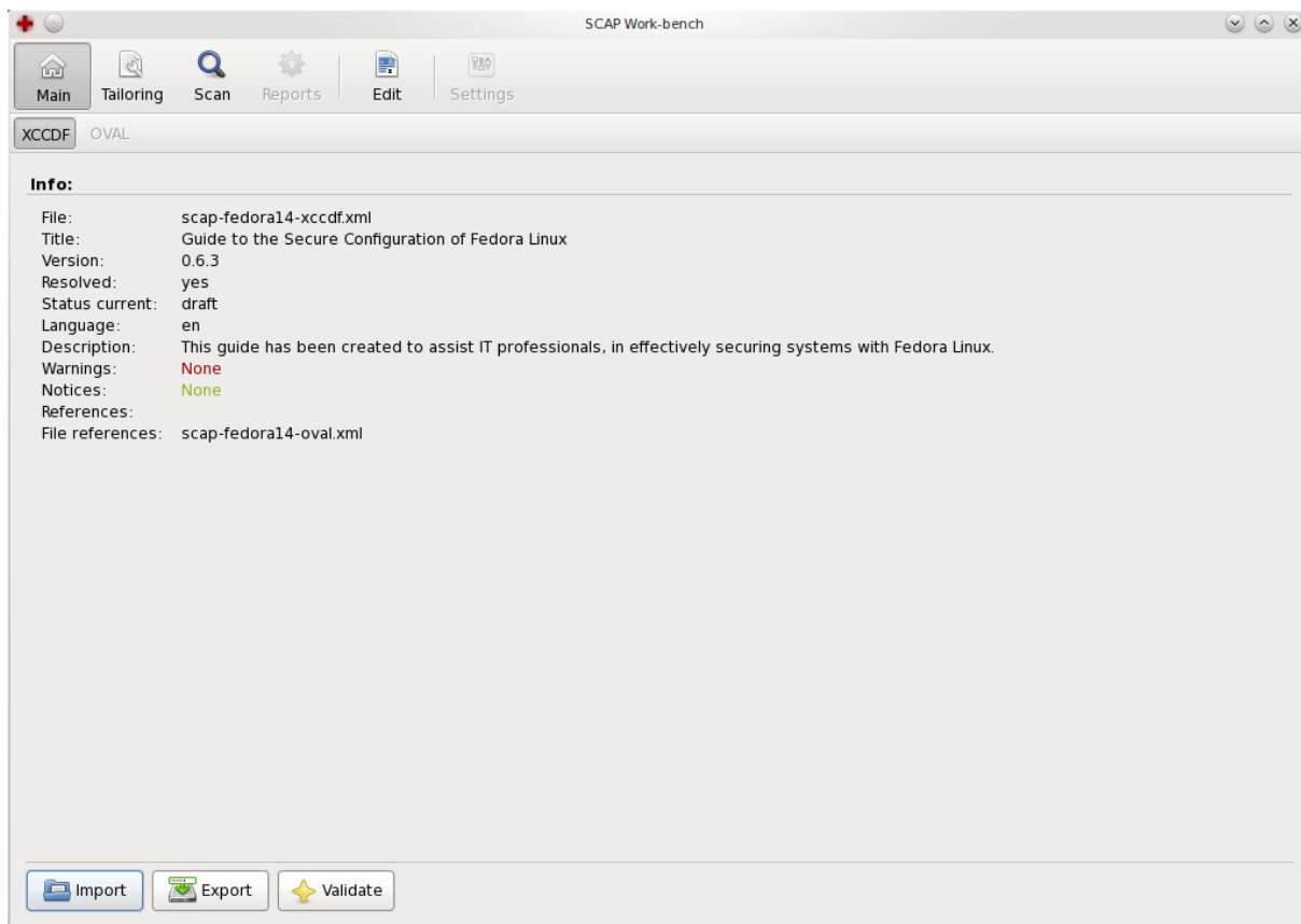
Obrázek 5.3: Hlavní okno
