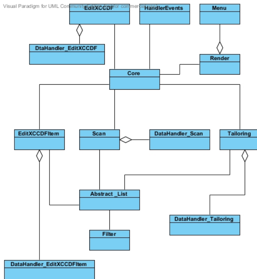
Obrázek 5.2: Diagram tříd
