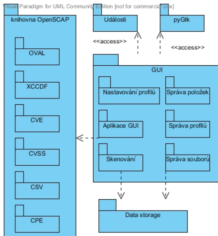
Obrázek 4.3: Analýza balíčků
