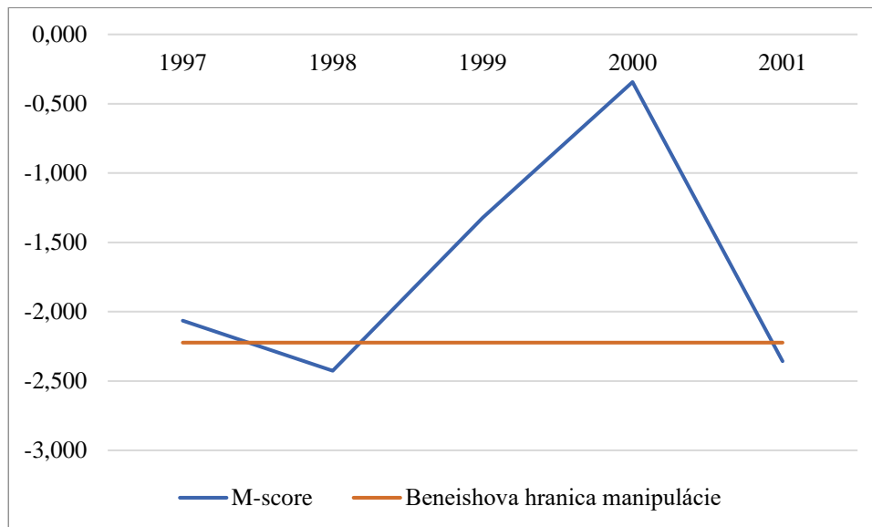
Graf 4: Výsledky Beneishovho modelu spoločnosti Enron
