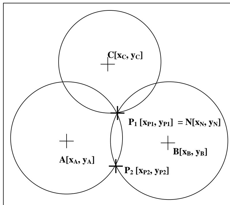
Obr. 2 Grafické znázornění algoritmu triangulace
