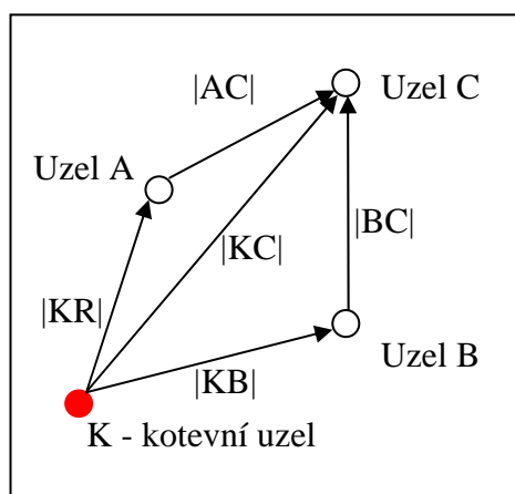
Obr. 6 Znázornění více cestního šíření lokalizační informace
