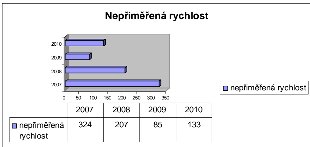
Graf č. 17 – Příčina nepřiměřená rychlost [11]
