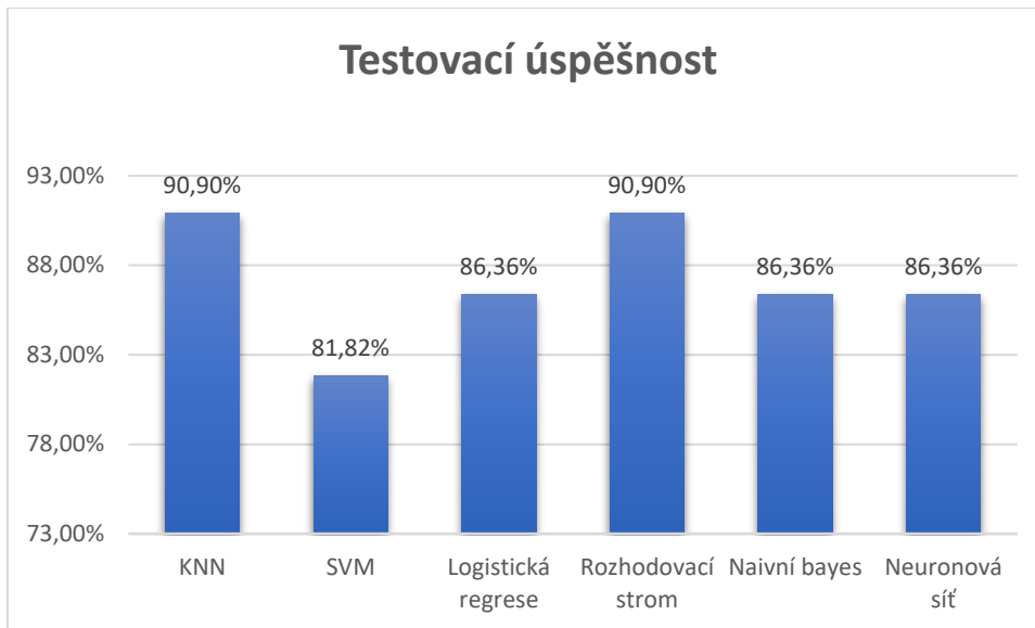
Obrázek 32 - Testovací úspěšnost vyladěných modelů
