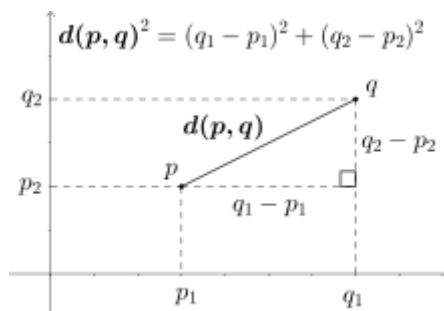
Obrázek 2- Euklidovská vzdálenost
