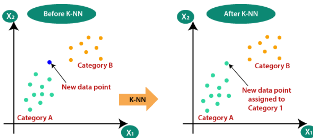
Obrázek 1 - KNN algoritmus
