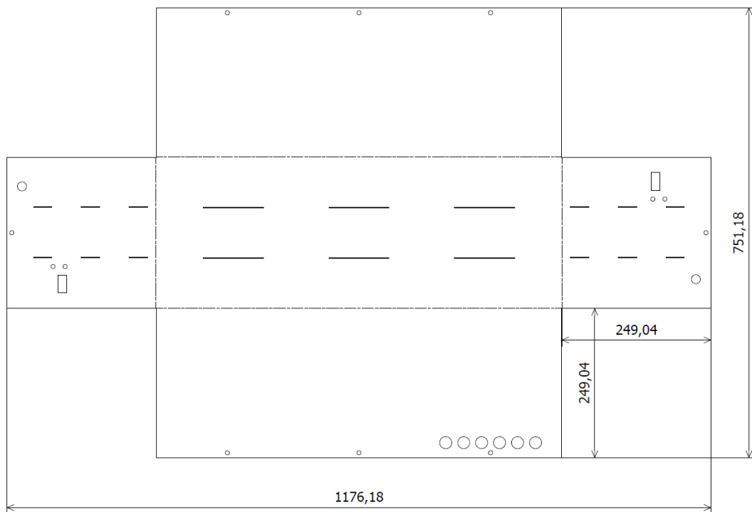
Obr. 52 Rozměry ohýbané součásti.
