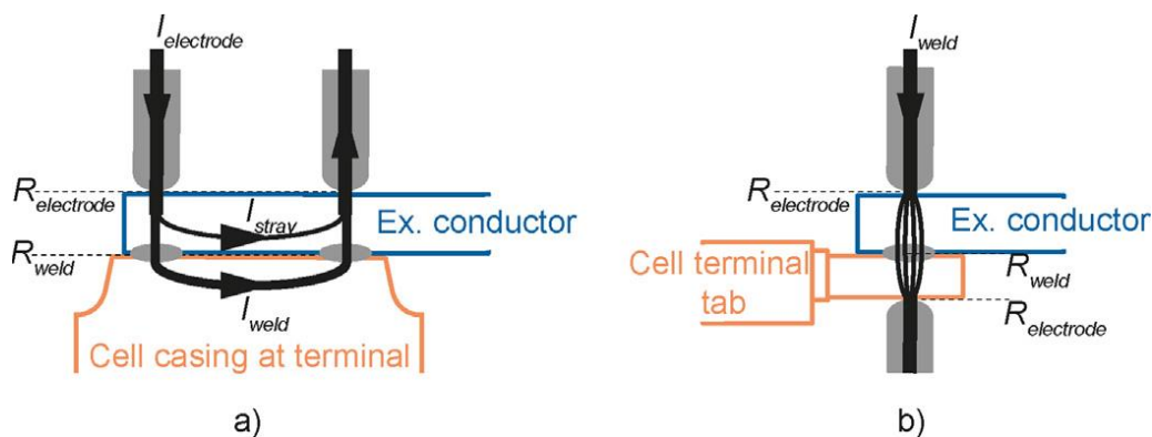
Obr. 8 Princip bodového odporového svařování za a) s paralelními elektrodami pro svařování cylindrických baterií a za b) pro svařování dvou plíšků pomocí elektrod oproti (například u Li-pol baterie) [21].
