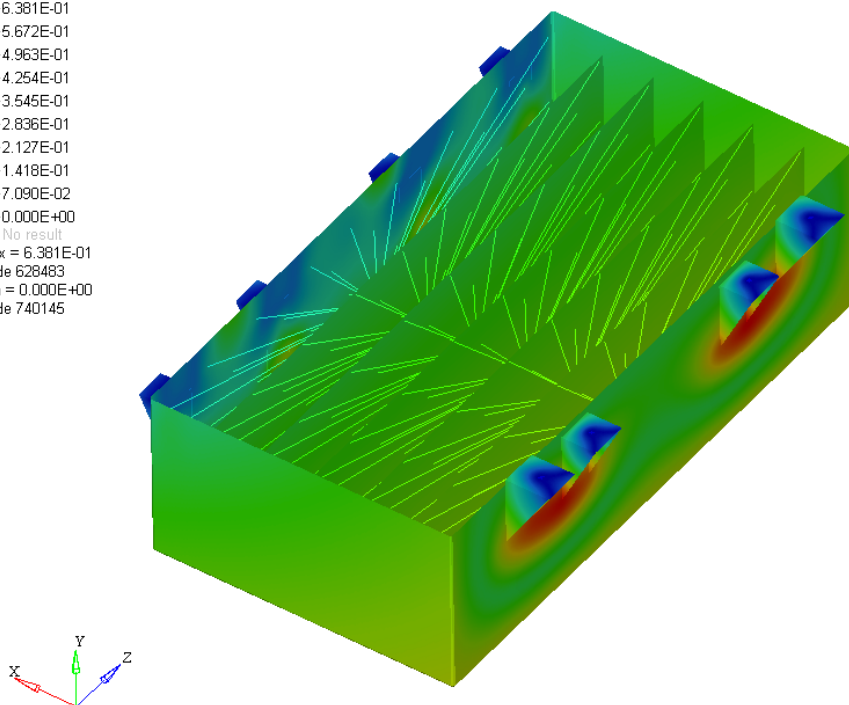
Obr. 74 Deformace boxu 3 při prudkém brždění.
