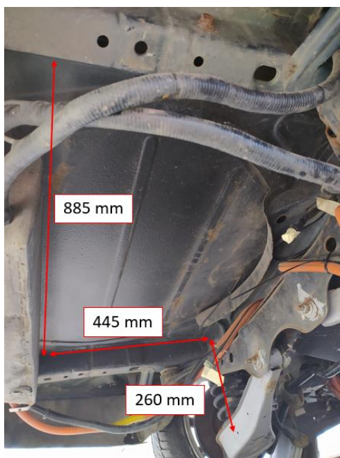
Obr. 39 Prostor pro rezervu, kde bude umístěný box 4.
