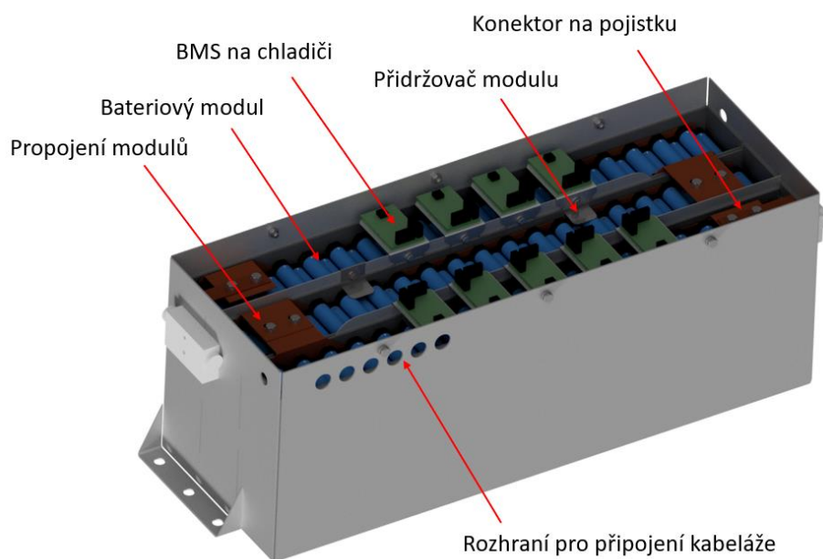
Obr. 59 Bateriový box 1 bez víka.
