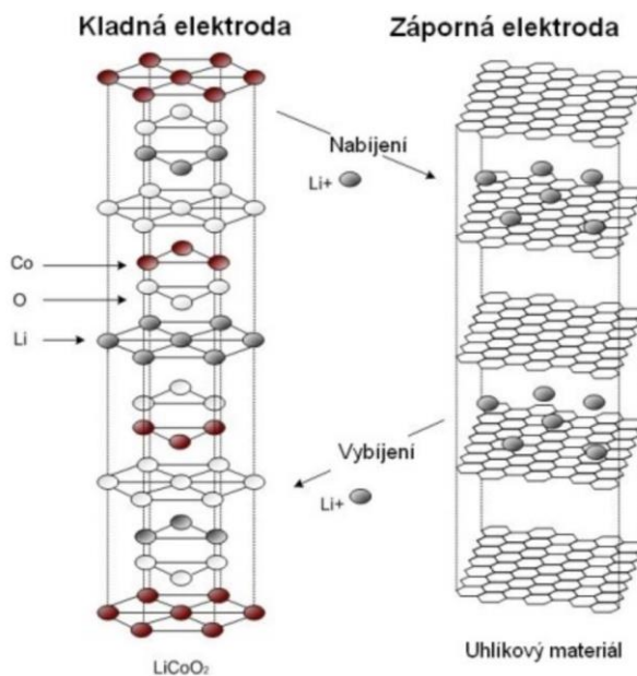
Obr. 2 Princip funkce lithium-iontové technologie [12].
