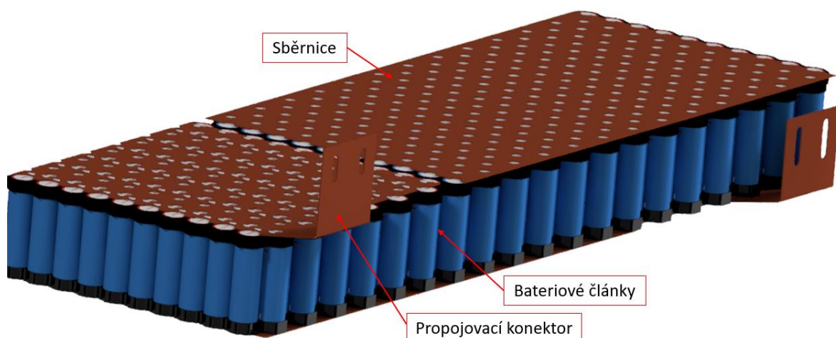
Obr. 44 Set tří modulů v zapojení 3s130p.
