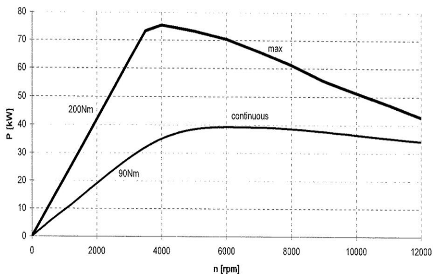
Obr. 33 Průběh výkonu motoru [38].
