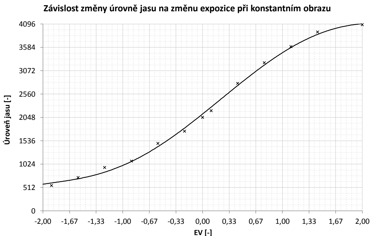
Obr. 18 Závislost změny úrovně jasu na změnu expozice při konstantním obrazu
