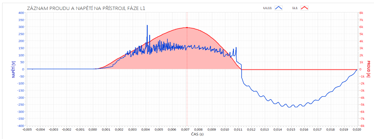
Obr. 20 Průběh napětí a proudu při vypínání zkratového proudu 7,5 kA
