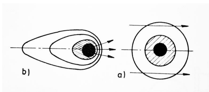
Obr. 4 Obloukový výboj v příčném řezu; a) v proudu vzduchu, b) pod vlivem magnet. pole [1]
