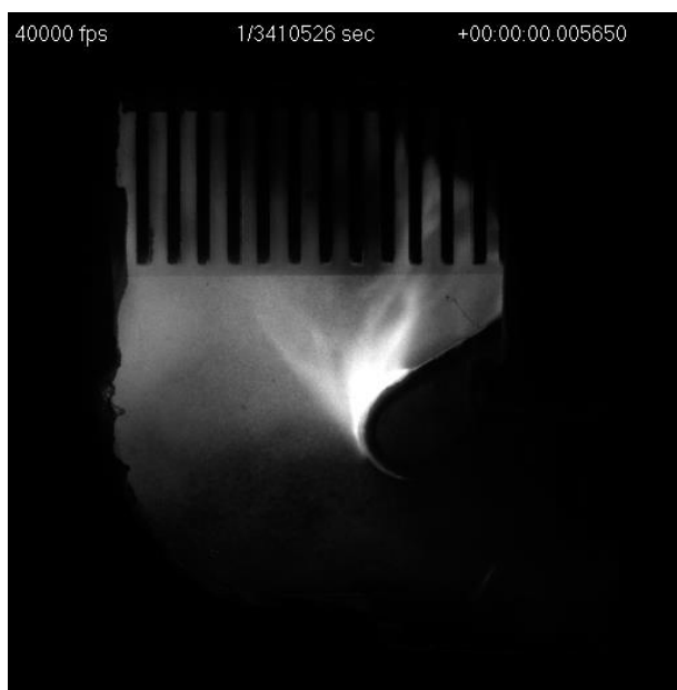
Obr. 23 Ekviintenzity el. oblouku pro snímek A
