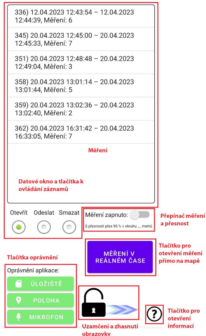
Obrázek 7: Rozložení obrazovky hlavní aktivity
