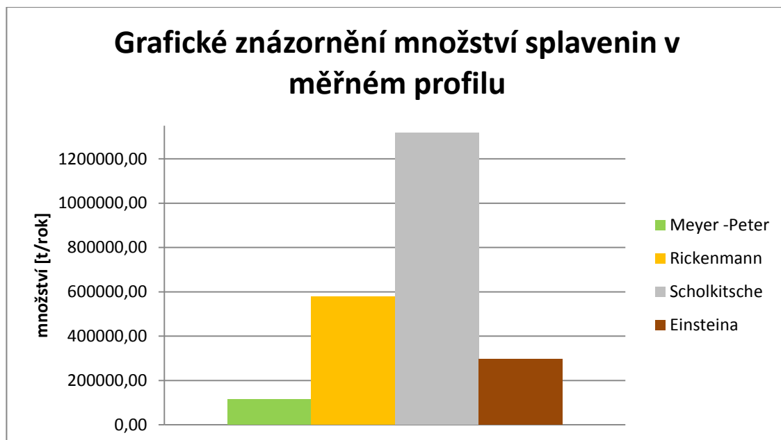
Graf 3 – Grafické znázornění množství splavenin
