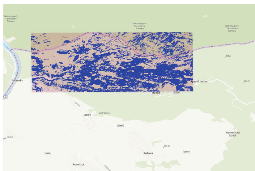
Obrázek 23 - výsledek klasifikace
