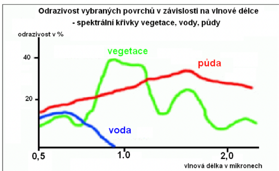
Obrázek 5 - odrazivost vybraných povrchů, zdroj [5 Svatoňová a kol.,]
