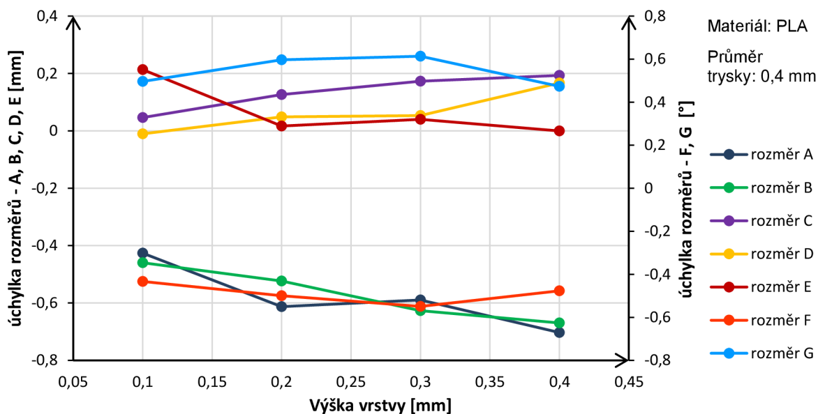
Obr. 5.17 Vliv výšky vrstvy na jednotlivé úchylky rozměrů – PLA.
