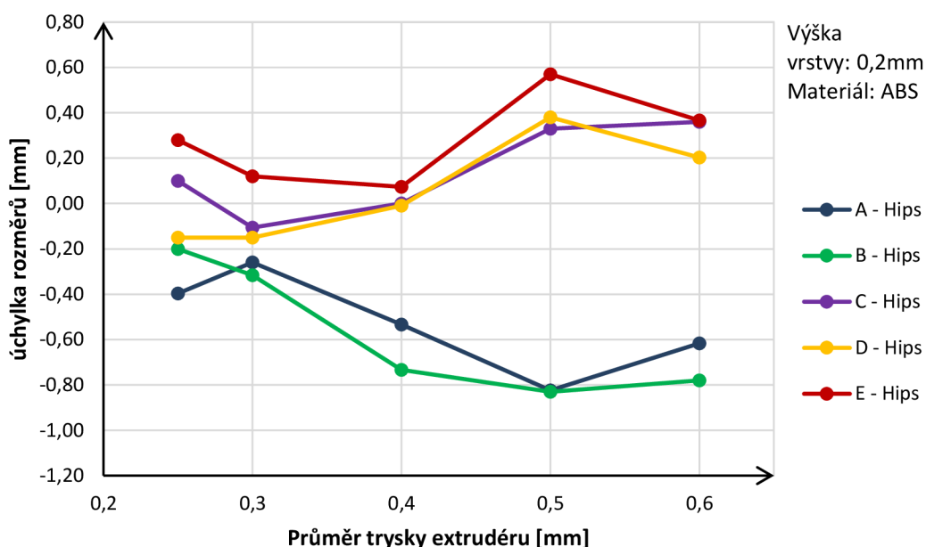
Obr. 5.16 Vliv průměru trysky extrudéru na jednotlivé úchylky rozměrů – Hips.
