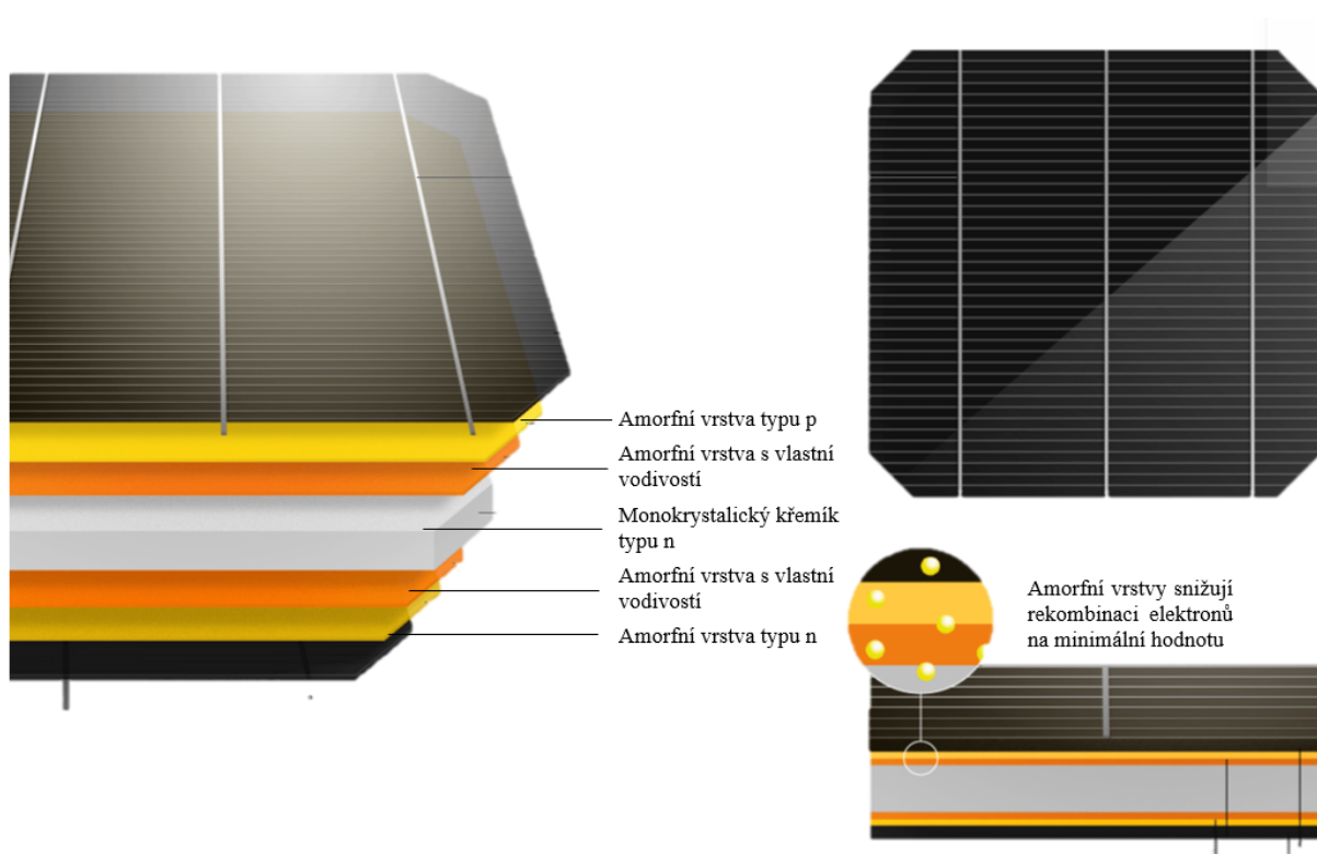
Obrázek 7: Hybridní články HIT (upraveno) [12].
