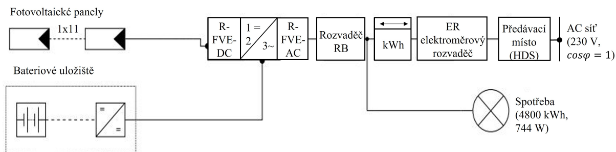
Obrázek 18: Elektroinstalace FVE.
