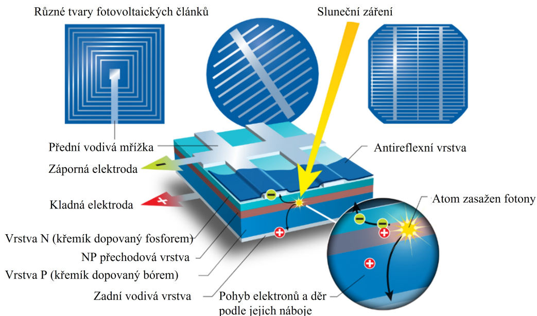
Obrázek 2: Přeměna energie v krystalickém křemíkovém solárním článku (upraveno) [6].
