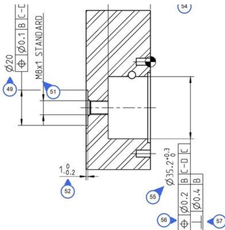
Obrázek 32 Výřez výrobního výkresu Zdroj: Inproma s.r.o.
