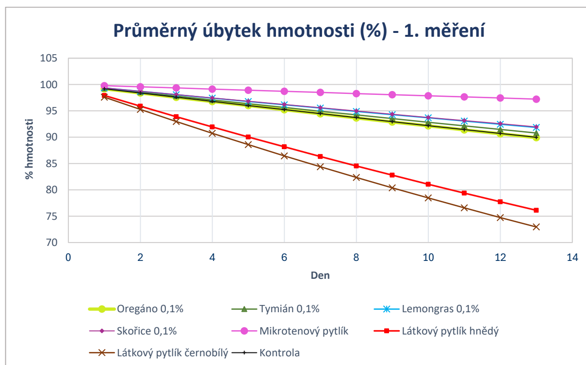
Graf 1: Průměrný úbytek hmotnosti vzorků v prvním pokusu (koncentrace 0,1 %)
