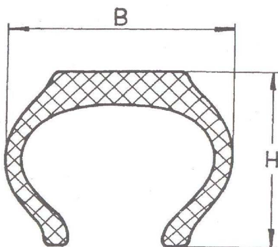
Obr. 18 značení pneu [11]
