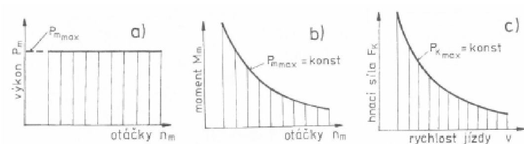
Obr 2 Ideální charakteristik[2]
