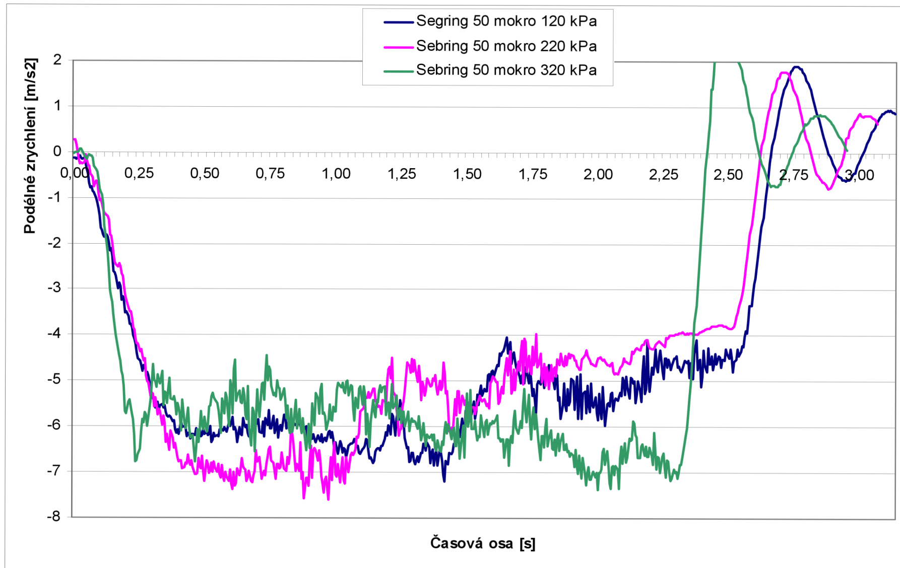
Obrázek 30 Porovnávací graf průběhu zpomalení, Sebring 205/55 R16 na mokrému povrchu
