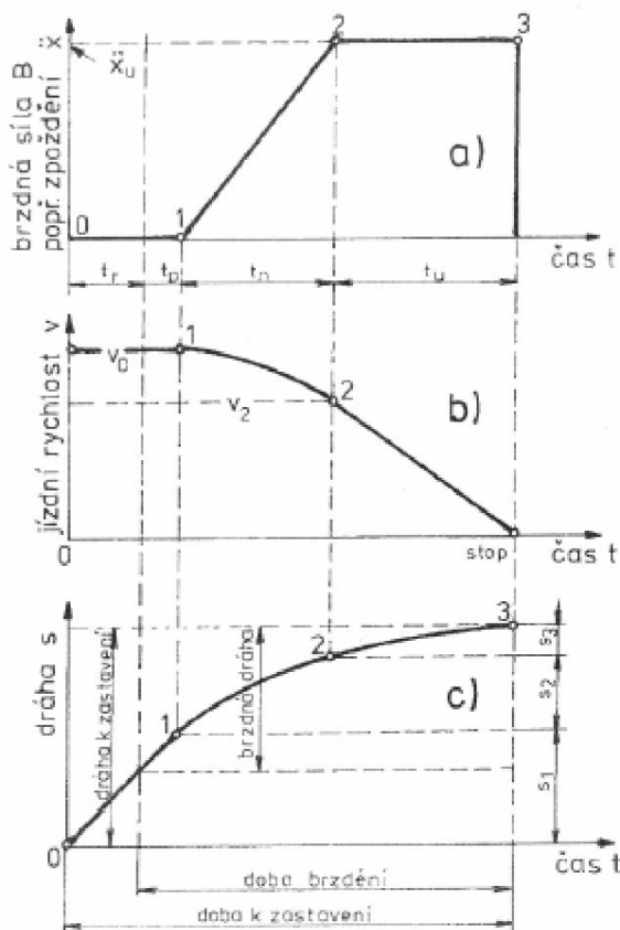
Obr. 11: Průběh brzdění[3]
