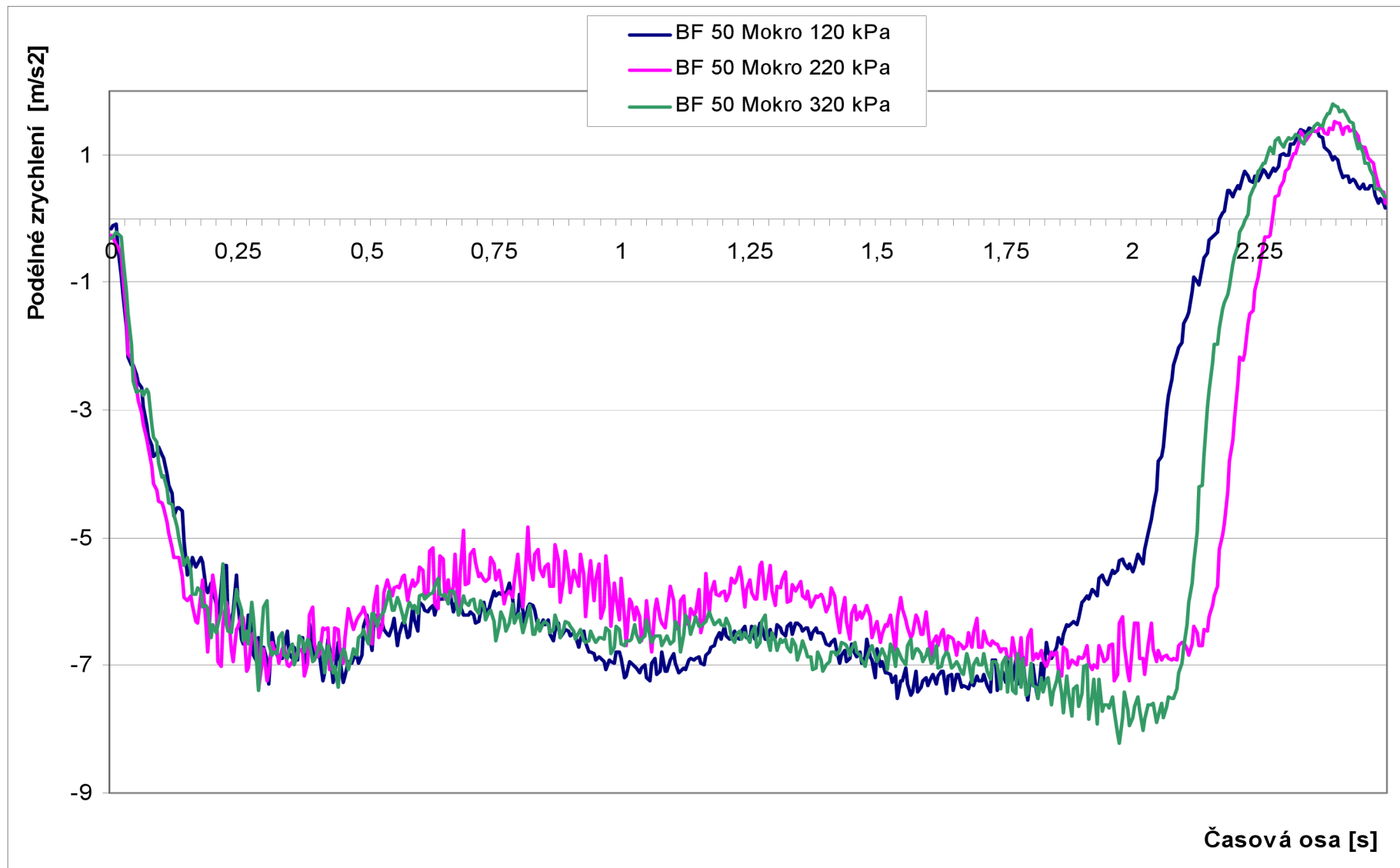
Obrázek 32 Porovnávací graf průběhu zpomalení, BF Goodrich 195/55 R15 na mokrém povrchu
