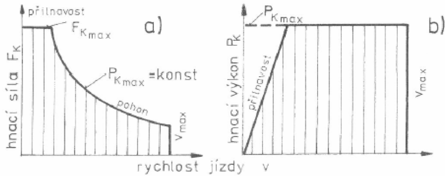
Obr. 5: Ideální rychlostní charakteristika pohonu vozidla omezená přilnavostí, maximální výkon a maximální rychlostí jízdy[3]
