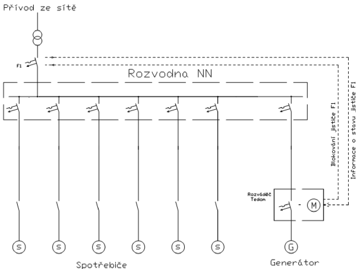
Obr 1-11 Kombinovaný provoz (P+I) [7]
