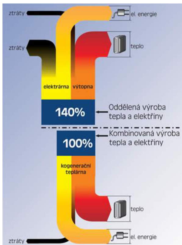
Obr. 1-6 Vyobrazení úspory paliva formou výroby elektřiny [15]
