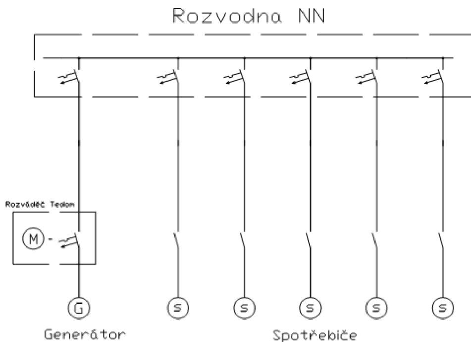
Obr. 1-9 Ostrovní provoz (I) [7]
