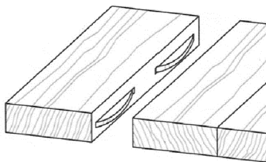
Obr. 4.5 Lamelový spoj[13]
