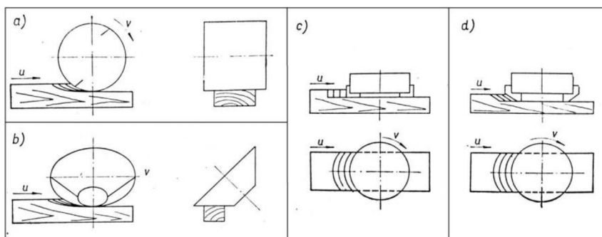
Obr. 5.2: Spôsoby frézovania [11]
