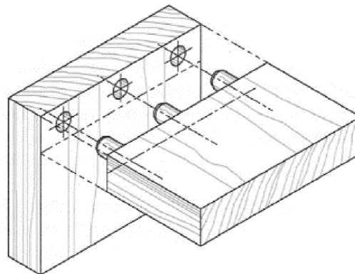
Obr. 4.4 Kolíkový spoj [13]
