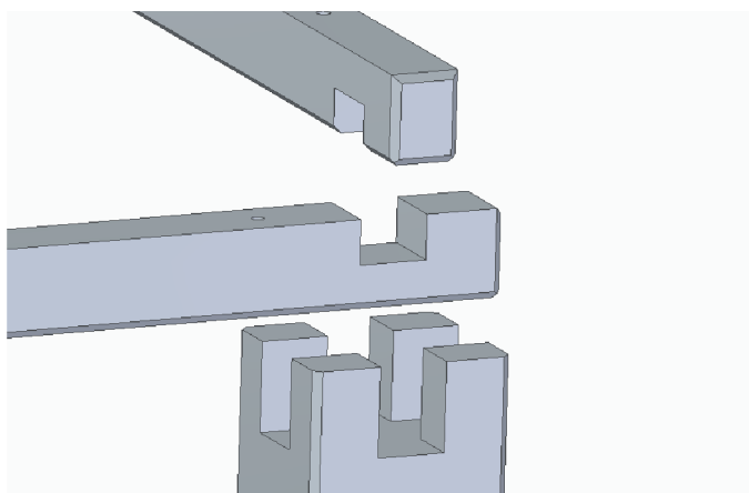
Obr. 4.6 Krížové preplátovanie
