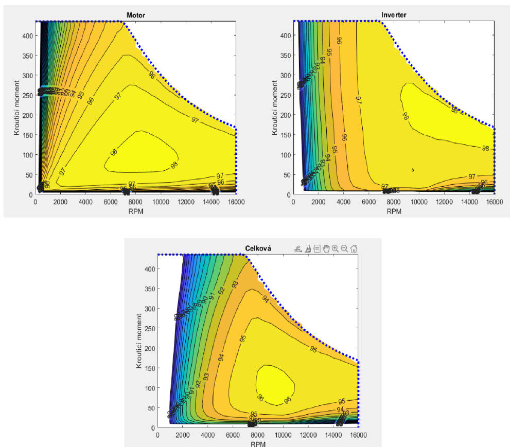
Obr. 21 - Účinnostní mapy
