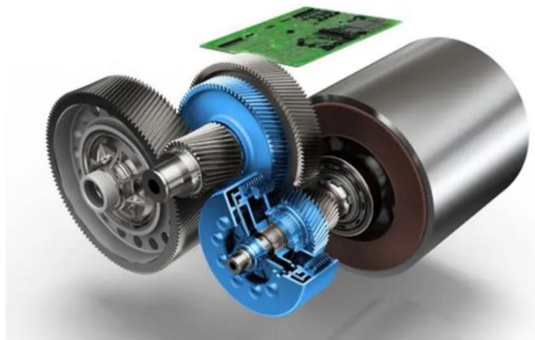
Obr. 12 - převodovka Tesla model X [40]
