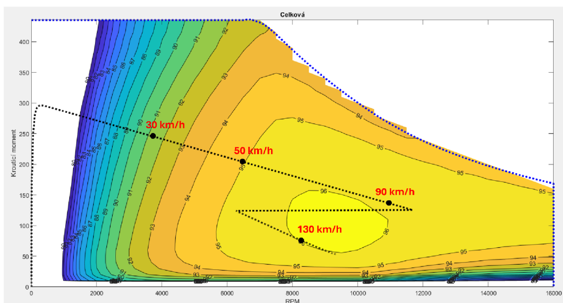
Obr. 25 - Účinnostní mapa pozvolné akcelerace s dvoustupňovou převodovkou
