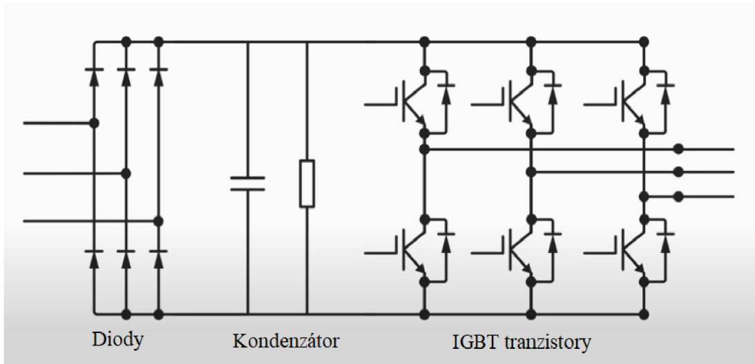
Obr. 8 - IGBT zapojení [26]
