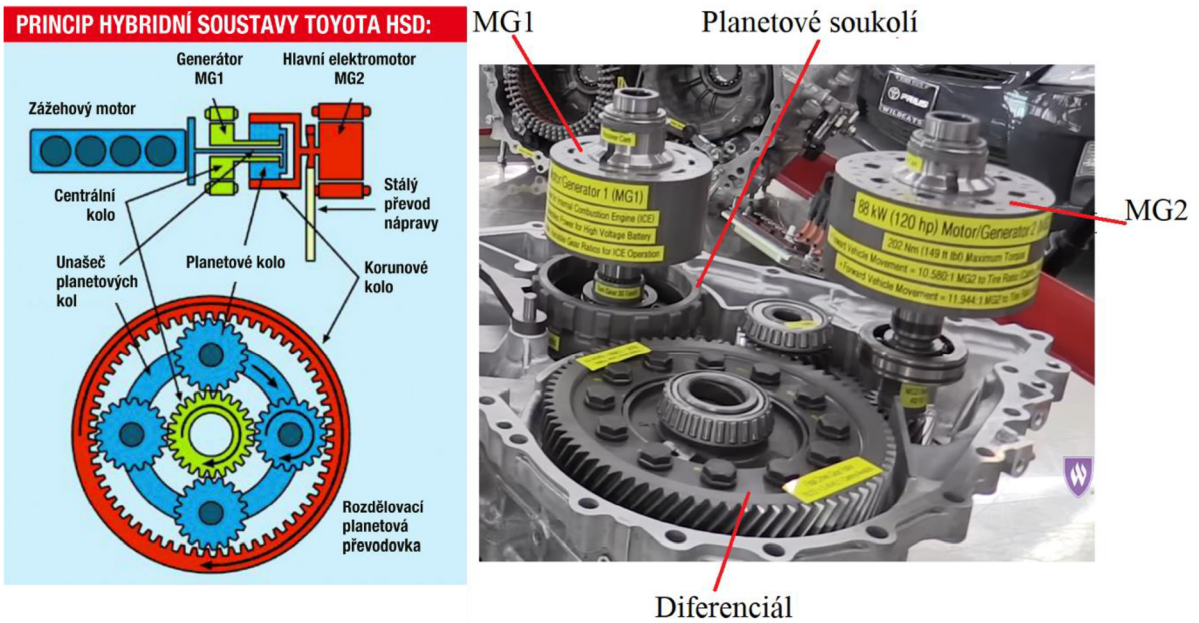
Obr. 16 – e-CVT převodovka [42] [48]
