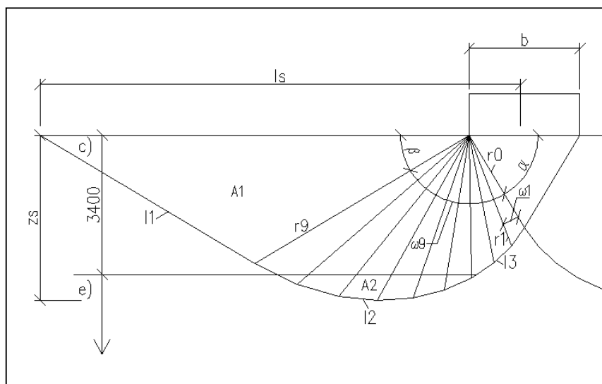
Obr. 8-23 Schéma pro výpočet průměrných charakteristik základové půdy
