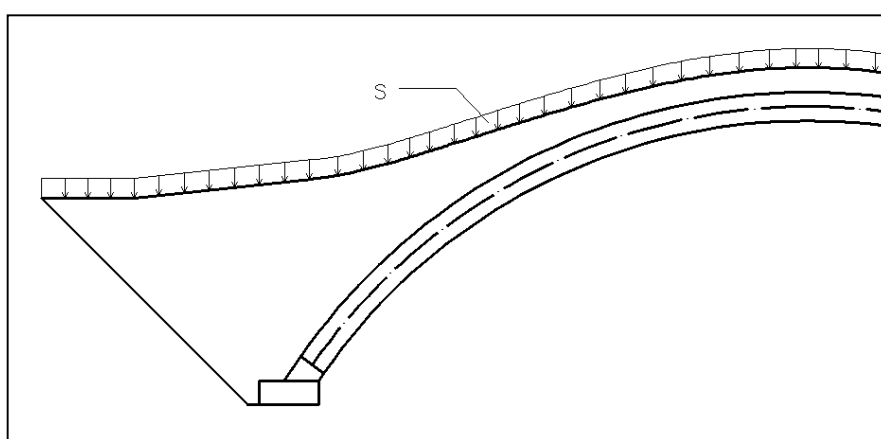
Obr. 8-6 Schematické zatížení terénu sněhem
