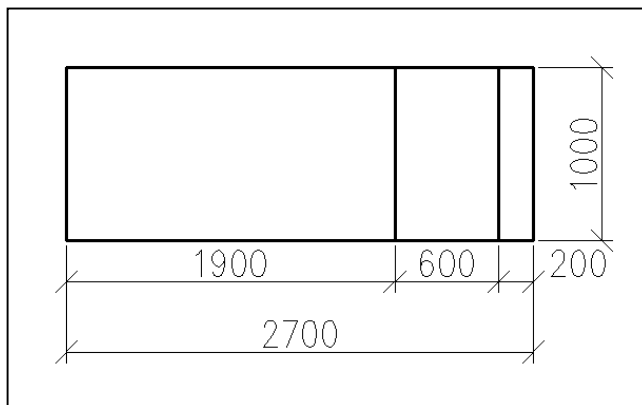
Obr. 8-19 Půdorysné schéma základového pasu – výpočtový model
