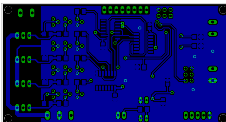
Ilustrace 9.2: Dolní strana DPS regulátoru
