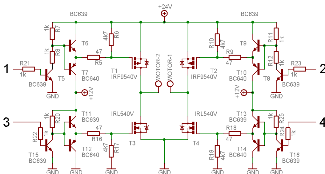
Ilustrace 4.4: Schéma výkonového stupně
