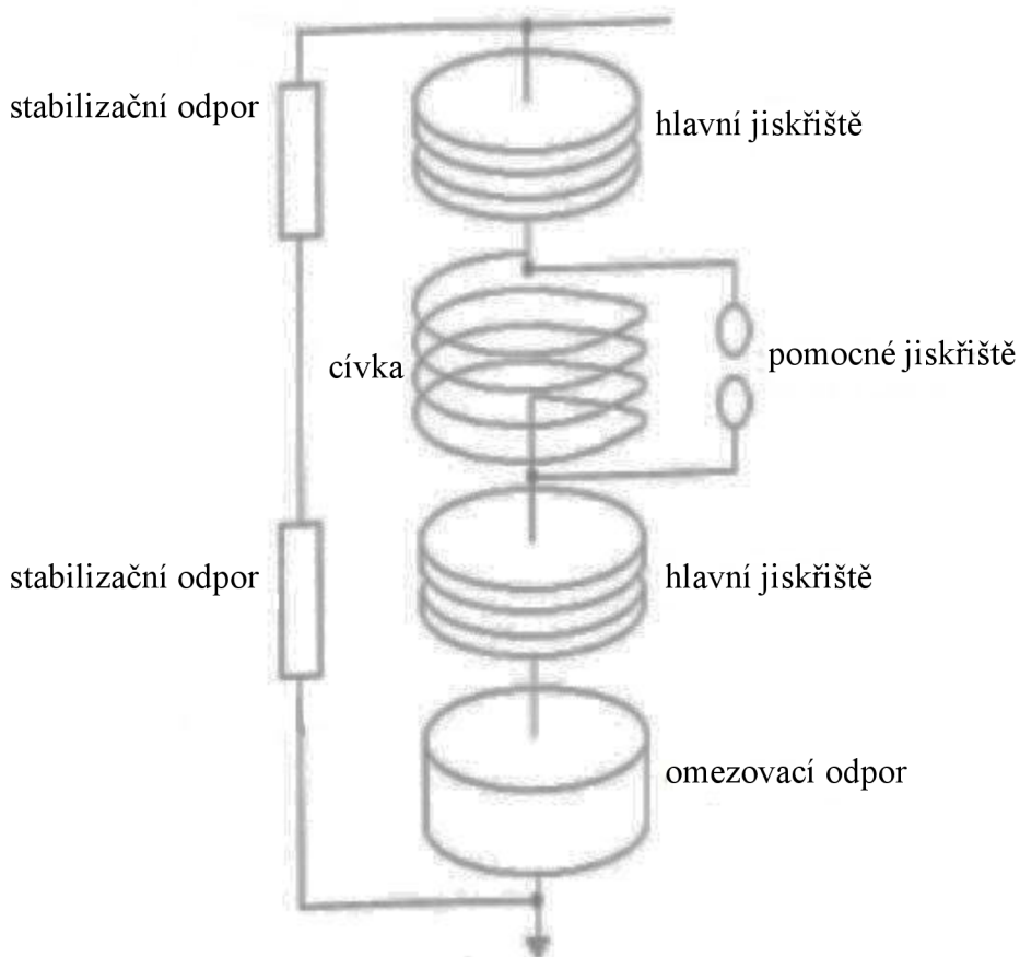
Obr. 4-6 Schéma složení ventilové bleskojistky – upraveno autorem [1]
