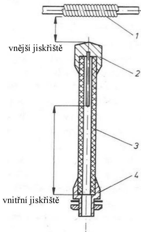
Obr. 4-4 Torokova trubice - upraveno autorem [5]
