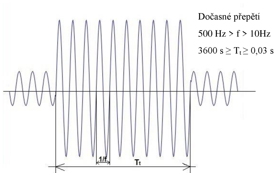
Obr. 3-2 Dočasné přepětí [1]
