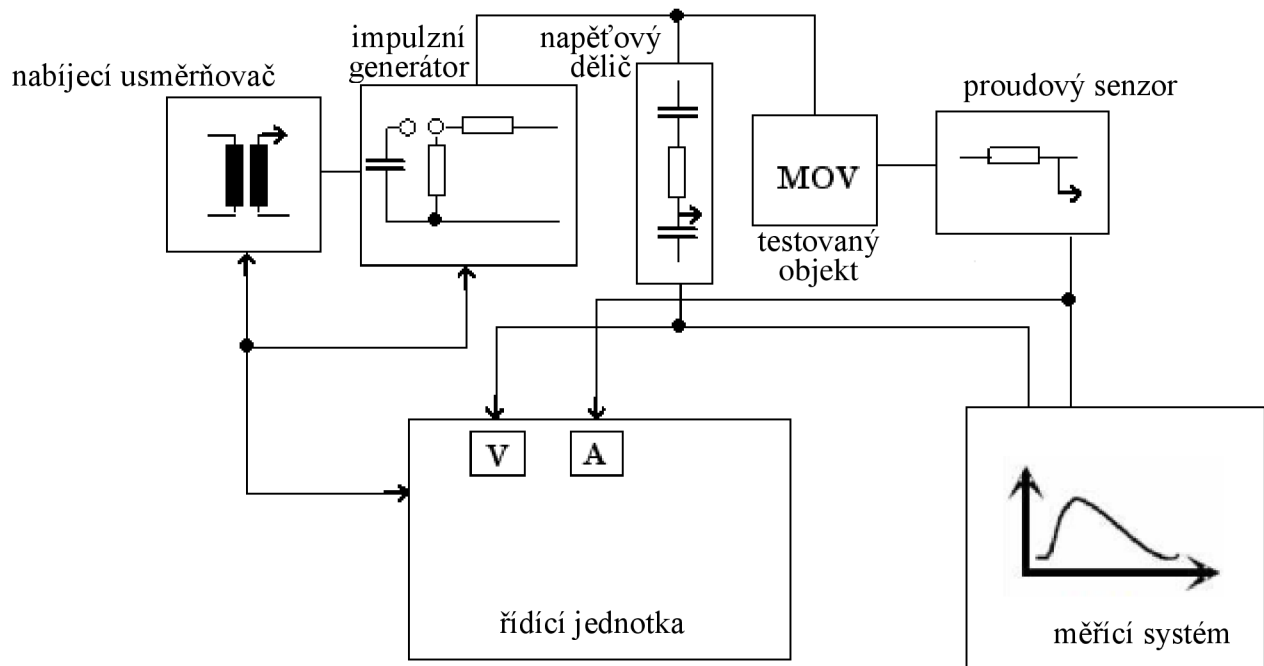
Obr. 7-3 Schéma zapojení
