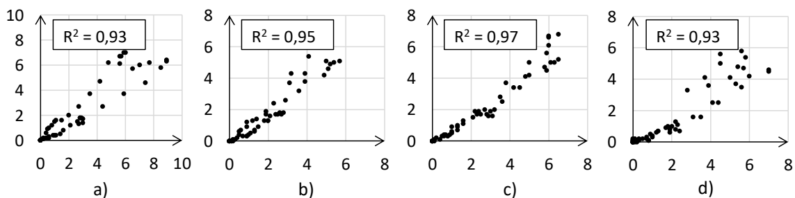
Obr. 5.14: Korelační diagramy interpolovaných hodnot s hodnotami srážkoměrů ČHMÚ. Stanice: a) Břevnov, b) Karlov, c) Vinohrady, d) Kbely. První etapa, srpen.
