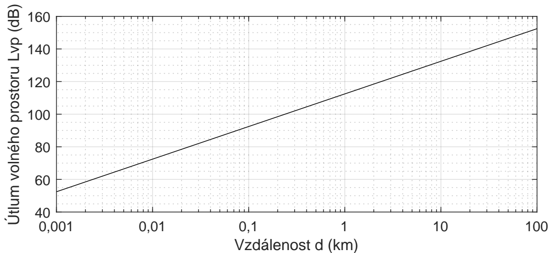
Obr. 3.1: Závislost útlumu L_{vp} ve volném prostoru na vzdálenosti d .
