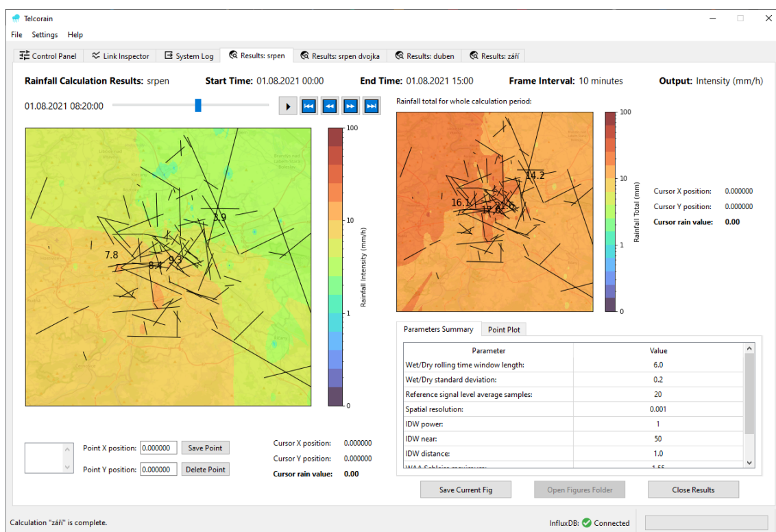
Obr. 6.7: Výstupní panel výpočtů aplikace Telcorain.
