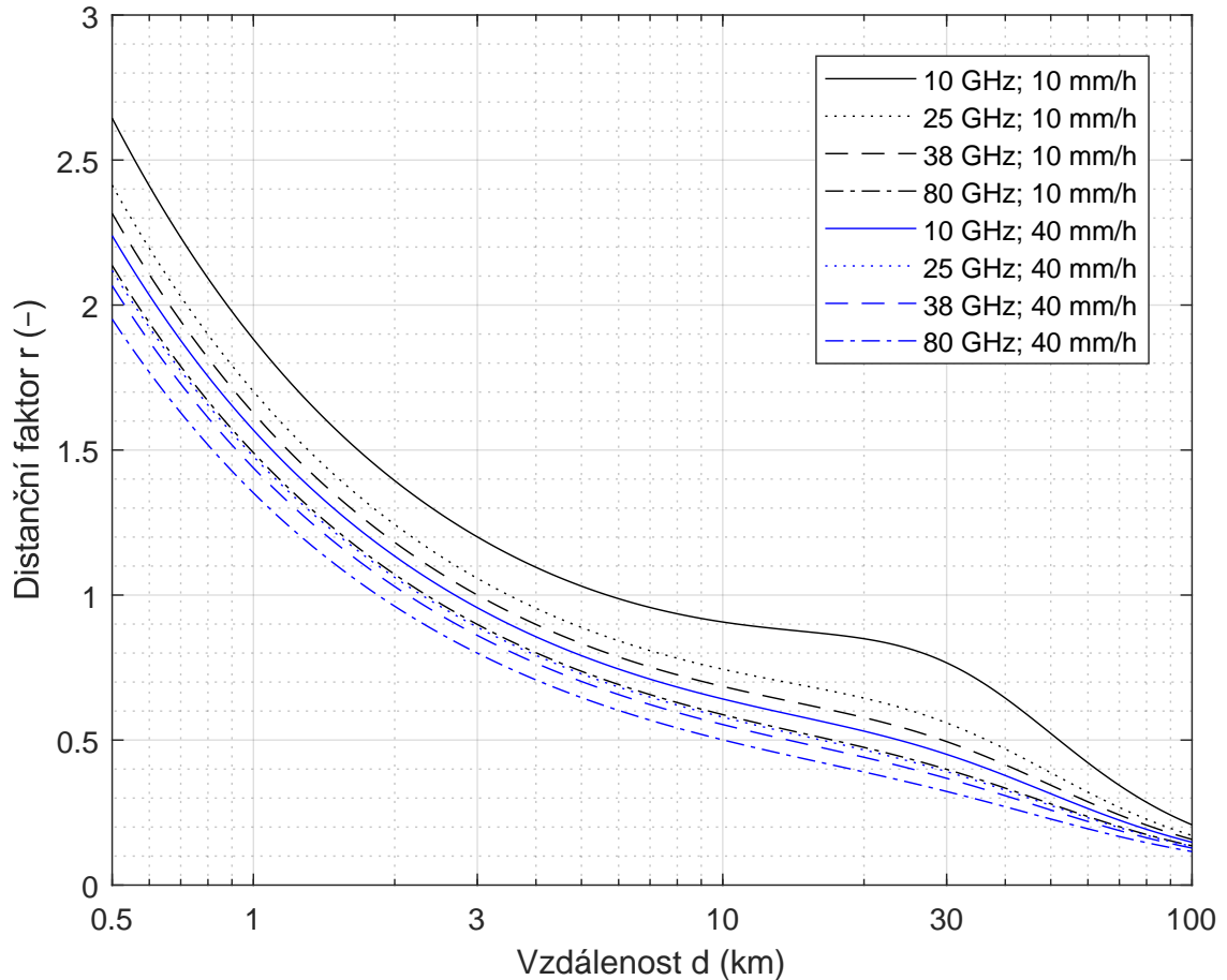
Obr. 3.9: Závislost hodnoty distančního faktoru r na délce spoje pro různé hodnoty frekvencí f a intenzity srážek R .
