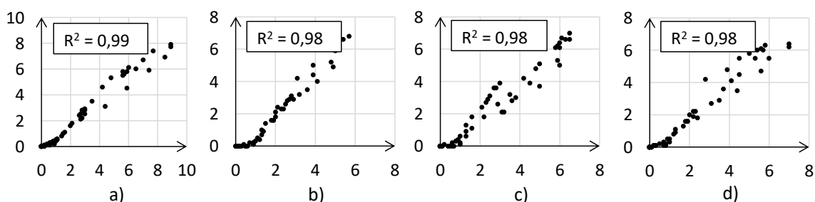
Obr. 5.20: Korelační diagramy interpolovaných hodnot s hodnotami srážkoměrů ČHMÚ. Stanice: a) Břevnov, b) Karlov, c) Vinohrady, d) Kběly. Druhá etapa, srpen.
