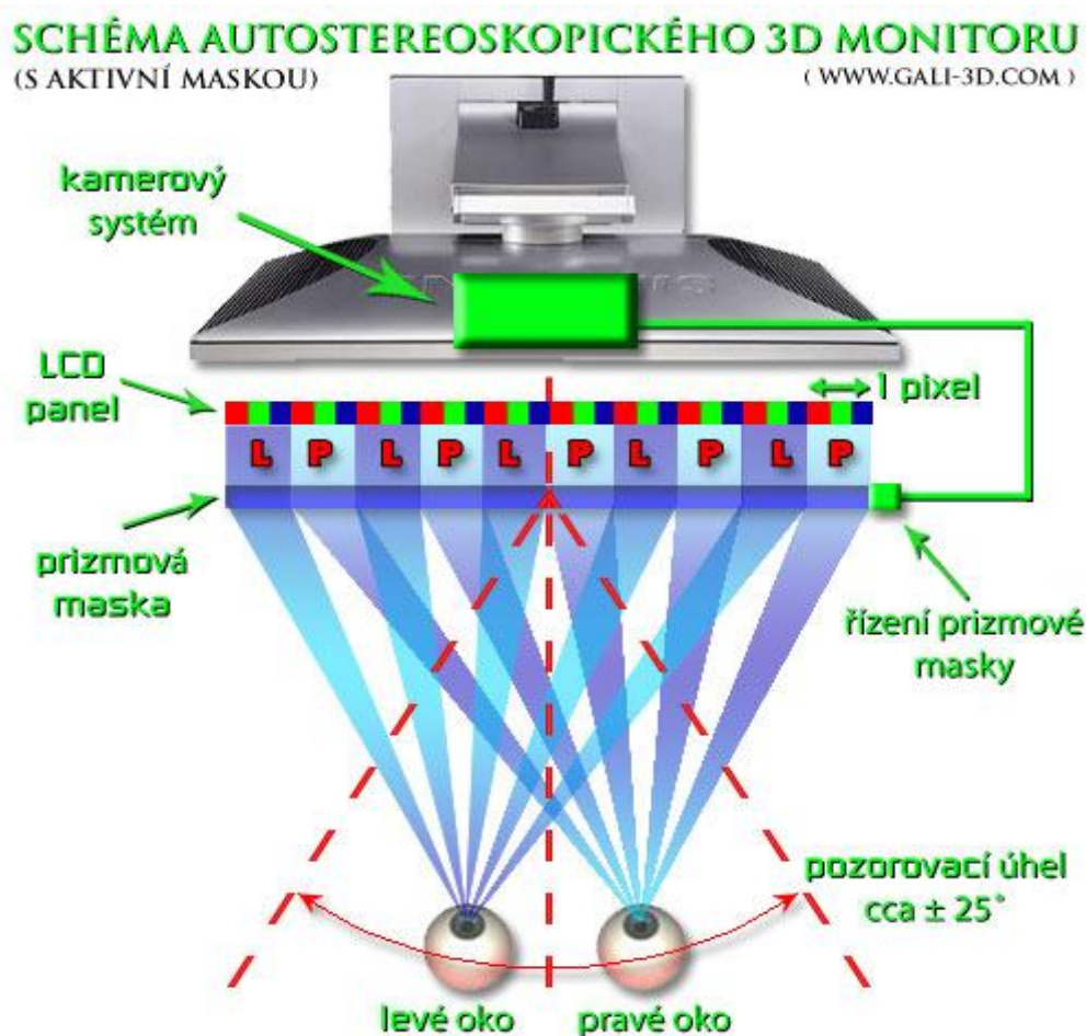
Obrázek 8: Autostereoskopická projekce(4)
