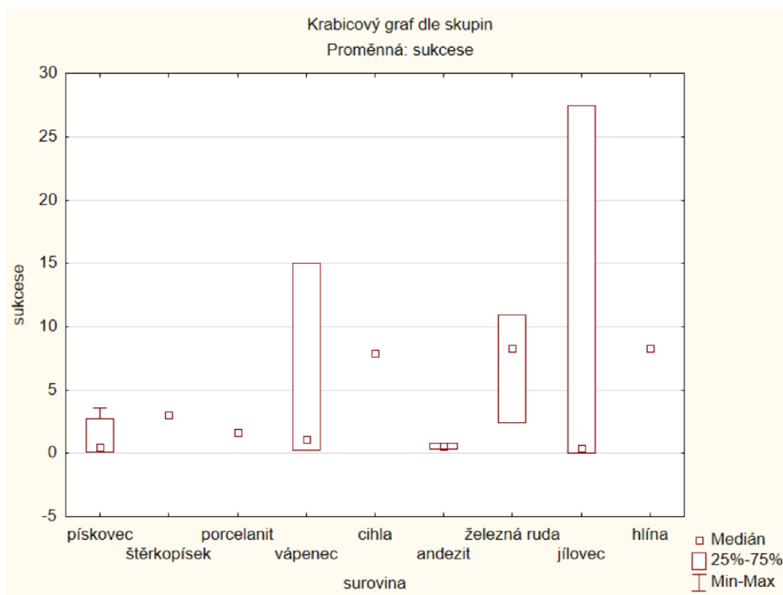
Obrázek č. 14 – Vztah vlivu těžené suroviny a sukcese – statistické vyhodnocení
