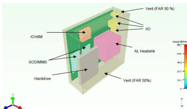
Obrázek 9 - Rozvržení komponent ve skříně - reference (6)
