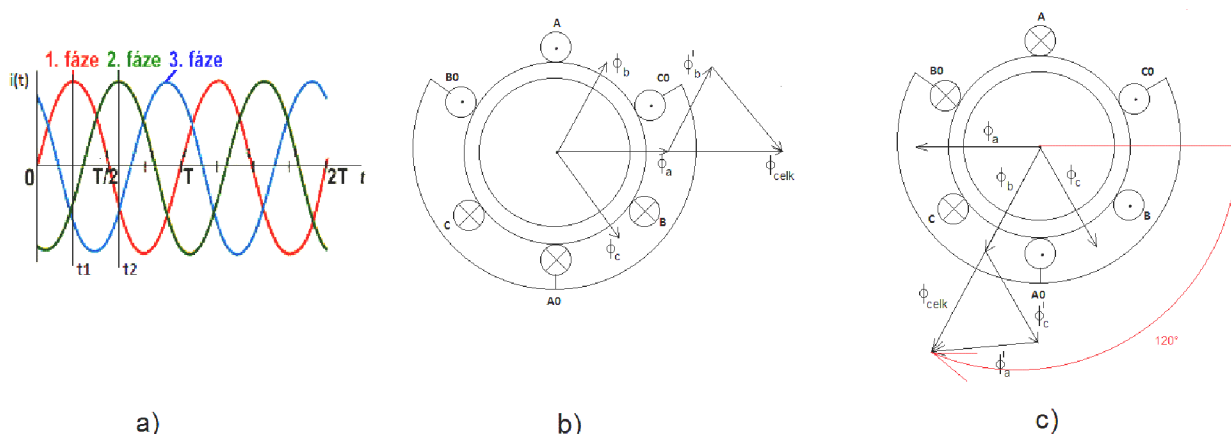
Obrázek 3: Časový průběh fázových proudů a směry proudů vinutími
