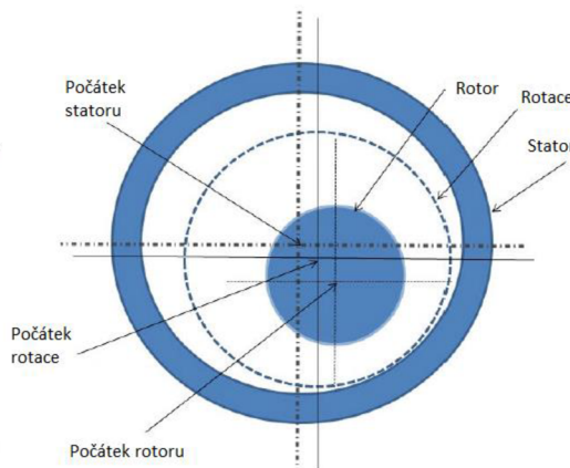
Obrázek 8: Kombinovaná excentricita
