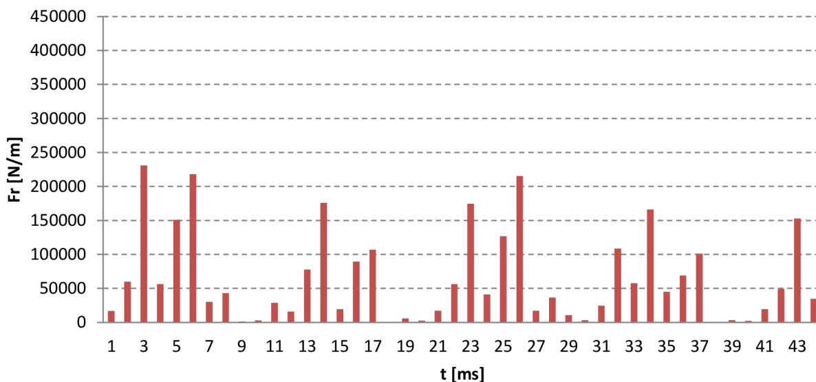
Obrázek 34: Velikost radiální síly v bodě -Y
