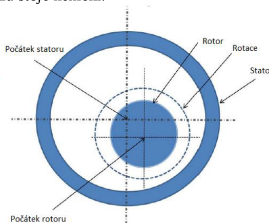
Obrázek 6: Statická excentricita
