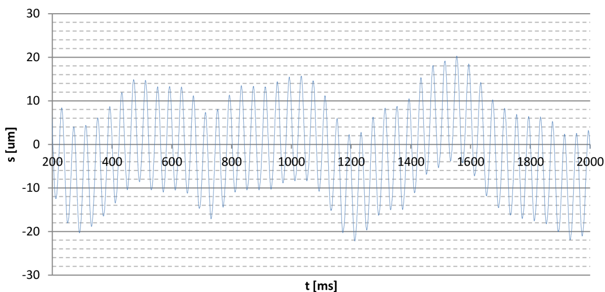
Obrázek 40: Průběh výchylky pro stroj se statickou excentricitou
