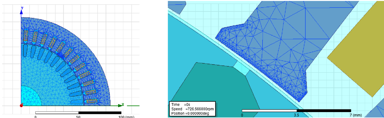
Obrázek 13: Síť meshe na jednotlivých částech motoru a jeho detail na zubu satoru
