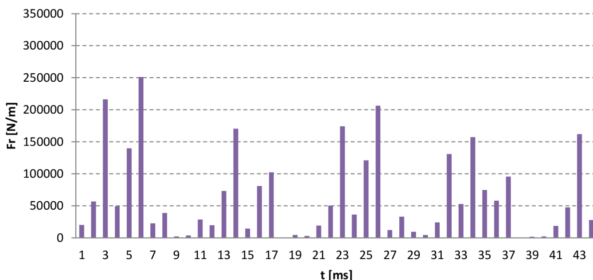
Obrázek 25: Velikost radiální síly v bodě -X
