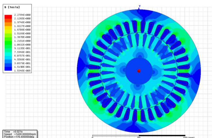
Obrázek 15: Rozložení magnetické indukce v motoru pro stroj bez poruchy
