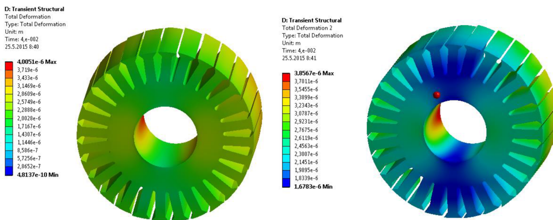
Obrázek 42: Výsledné rozložení deformace pro celý stroj a pouze rotor
