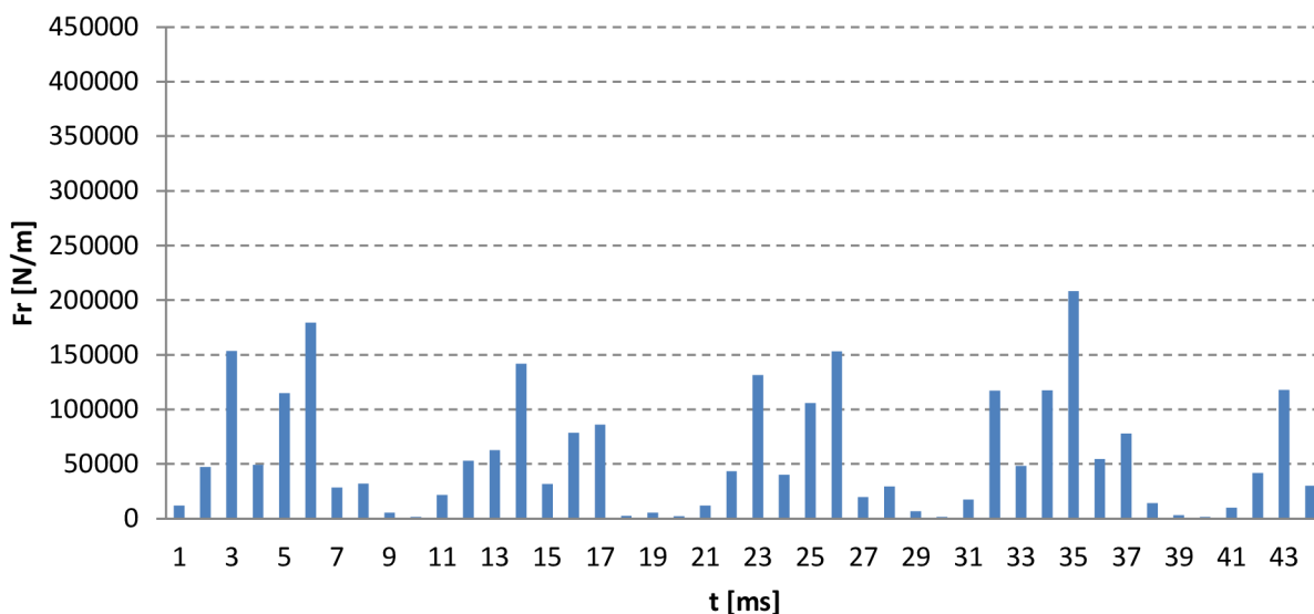
Obrázek 33: Velikost radiální síly v bodě +X
