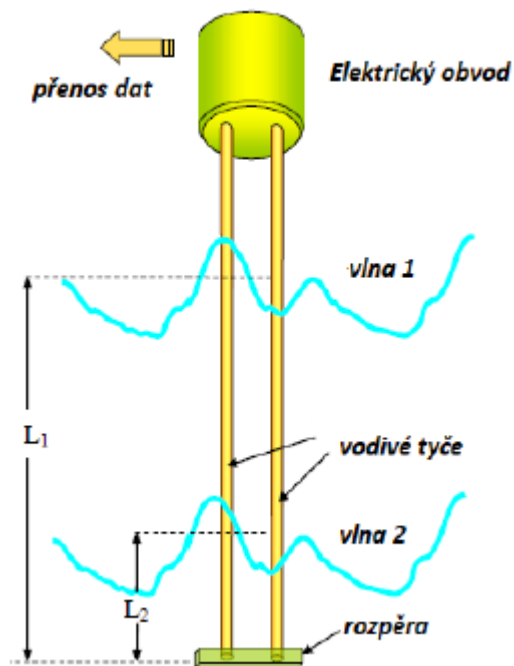
Obr. 7 Odporový snímač [10]
