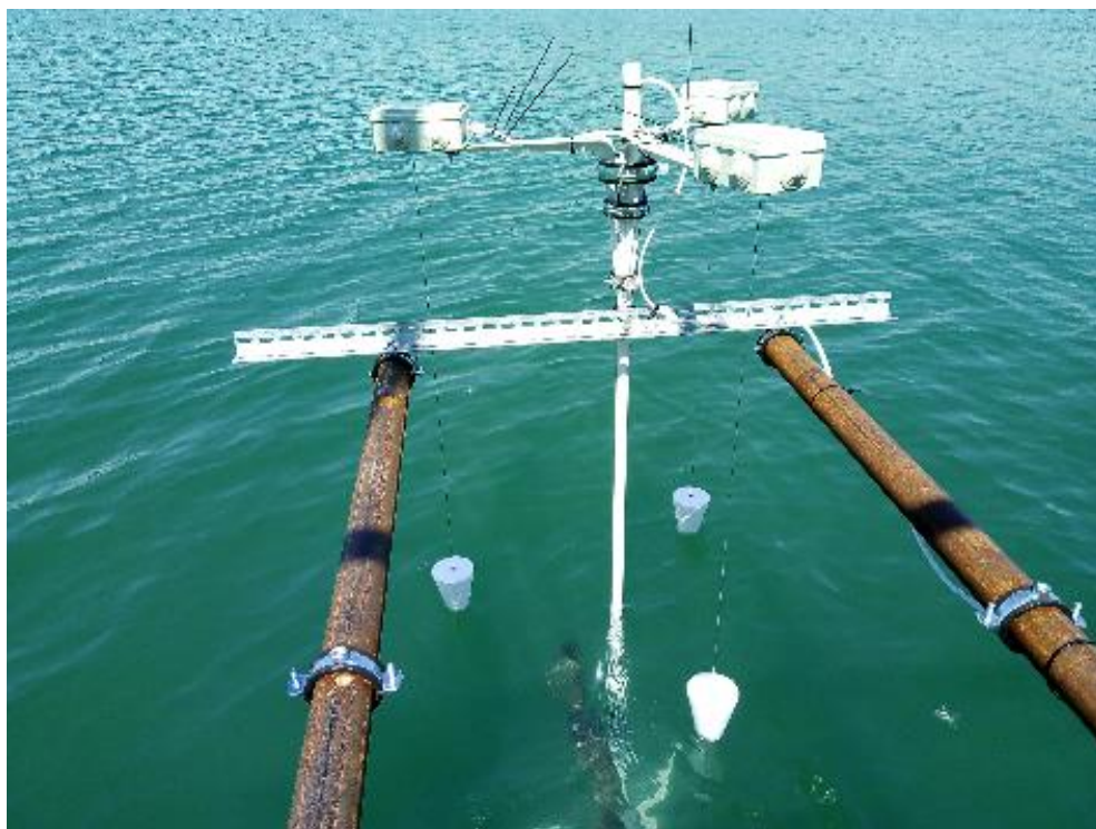
Obr. 14 Čidla pro snímání pohybu hladiny [18]
