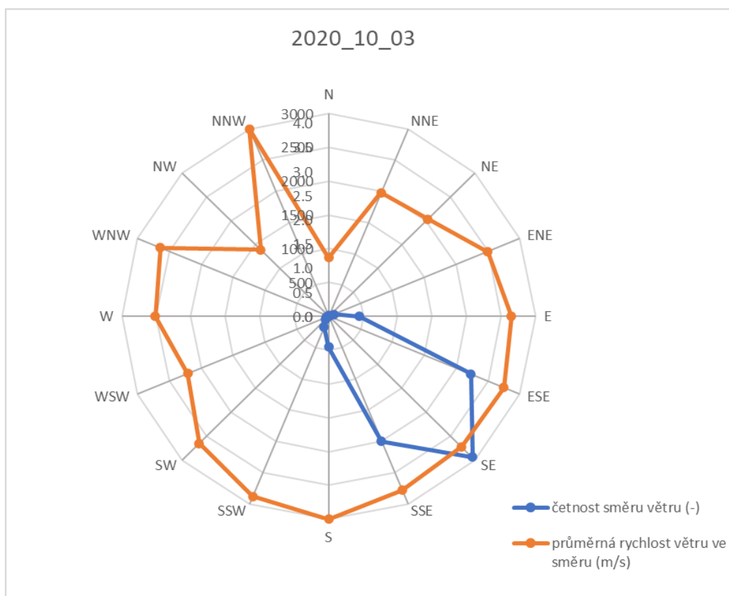
Obr. 46 Vyhodnocení anemometru
