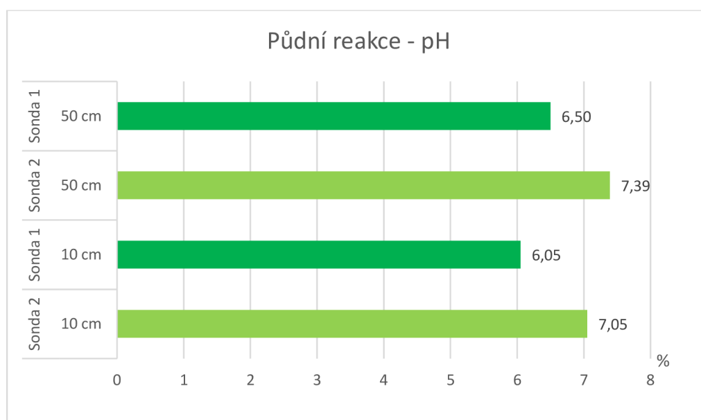
Obrázek 30: Graf výsledků půdní reakce pH laboratorních rozběrů odebraných půdních vzorků
