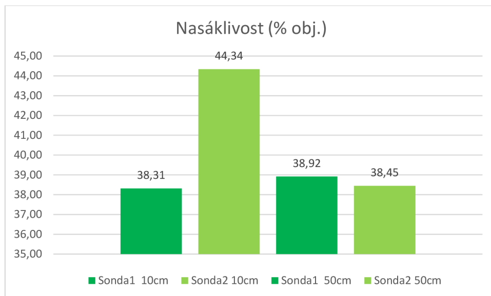
Obrázek 18: Graf výsledků nasáklivosti laboratorních rozborů odebraných půdních vzorků. Hodnoty získané z jednotlivých sond jsou barevně odlišeny.
