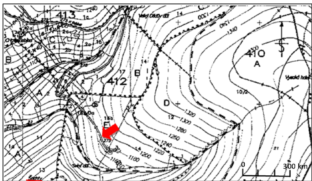
Obr. 8. Výšeč lesní mapy s lokalizací nového výskytu páskovaných magnetitových rud (silná červená šipka). Staré důlní dílo „Mniší jámy“ je na mapce označeno jako „Šachty“ (červeně podrženo) (Kopa a Fojt 2003).
