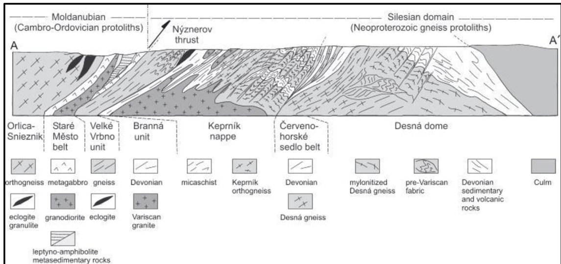
Obr. 5. Geologický řez silezikem zobrazující stavbu a litologii jednotlivých jednotek a hlavní tektonické hranice (Košuličová a Štípská 2007).
