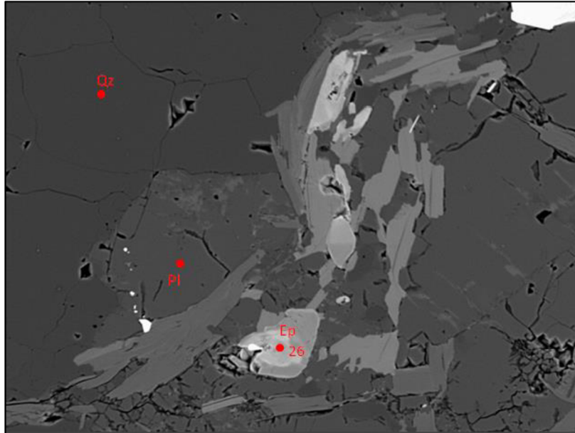
Obr. 27. Epidotové zrně v křemen-magnetitové rudě. Na snímku je viditelné také akcesoricky se vyskytující plagioklas. Vzorek VER-PB-19. BSE snímek. Šířka snímku 0,25 mm. Foto: P. Gadas
