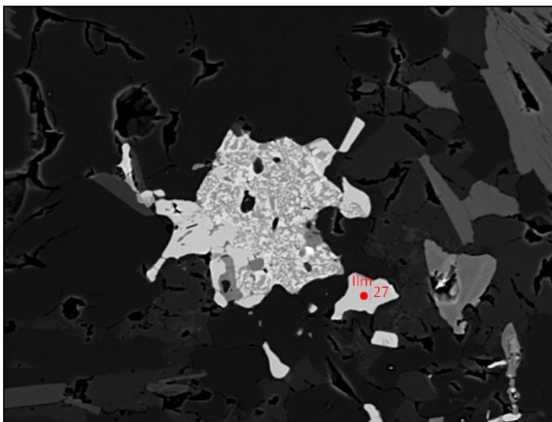
Obr. 29. Uprostřed snímku, vedle malých ilmenitových zm, je agregát složený z \text{TiO}_2 -minerálu (tmavý) a Fe-oxidu (téměř bílý). Patrně jde o výsledek rozpadu pevného roztoku (titanomagnetit nebo ilmenoheematit). Z analýzy vyplývá, že tento agregát nemůže být výsledkem přeměny titanitu, jelikož nebyla nalezena přítomnost Ca. Vzorek VER-PB-19. BSE snímek. Šířka snímku 0,15 mm. Foto: P. Gadas
