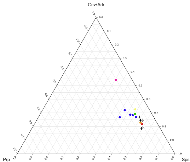
Obr. 46. Pozice granátů v systému Prp – Sps – Grs+Adr. Černé křížky zobrazují pozice analyzovaných granátů z lokality Pod Břidličnou. Barevná kolečka jsou analyzované granáty z lokality Kosaře-Špičák.
