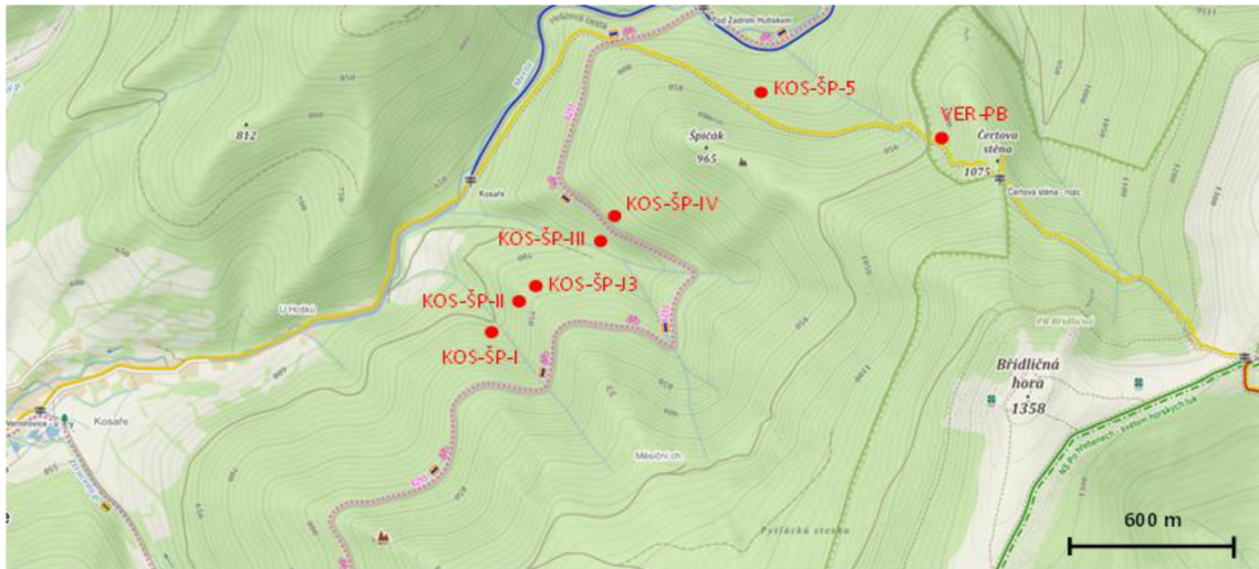
Obr. 12. Zaznačené navštívěné lokality v okolí Vernířovic. Vernířovice – Pod Břidličnou (VER-PB), Kosaře – Špičák – štola 5 (KOS-ŠP-5), Kosaře – Špičák – štola IV (KOS-ŠP-IV), Kosaře – Špičák – štola III (KOS-ŠP-III), Kosaře – Špičák – štola II (KOS-ŠP-II), Kosaře – Špičák – štola I (KOS-ŠP-I). Zdroj: Mapy.cz ( https://mapy.cz/turisticka?l=0&x=17.1667264&y=50.0359057&z=15 ).
