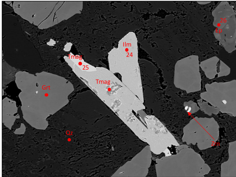
Obr. 38. Lištovité průřezy dvěma tabulkami ilmenitu obsahujícími uzavřeniny titanomagnetitu (ilmenohepatitu) místy s odměšeninami \text{TiO}_2 . V okolí je viditelné i drobné zrno zirkonu a zrno chemicky zonálního epidotu. Vzorek KOS-ŠP-II-5. BSE snímek. Šířka snímku 0,3 mm. Foto: P. Gadas
