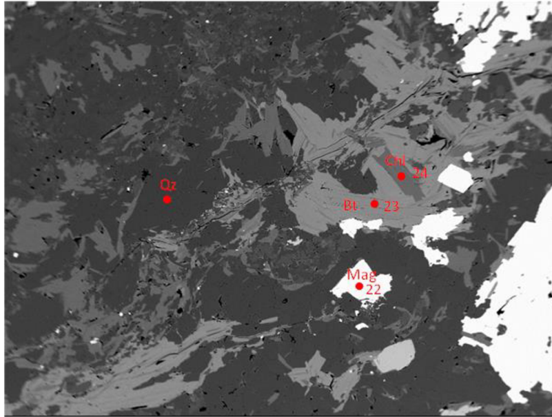
Obr. 25. Biotit obklopující šupinu chloritu v křemen-magnetitové rudě. Vzorek VER-PB-19. BSE snímek. Šířka snímku 2,2 mm. Foto: P. Gadas
