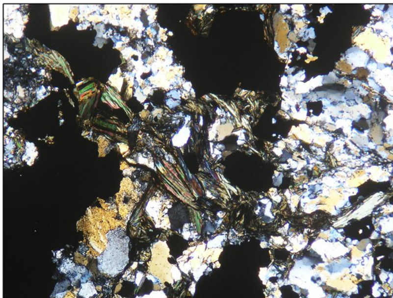
Obr. 24. Detail šupinek biotitu, v některých partiích již plně chloritizovaného, což lze vidět ve středu snímku (anomálně modrá, jindy hnědá interferenční barva). Vzorek VER-PB-25. Leštěný výbrus, XPL. Šířka snímku 2 mm.
