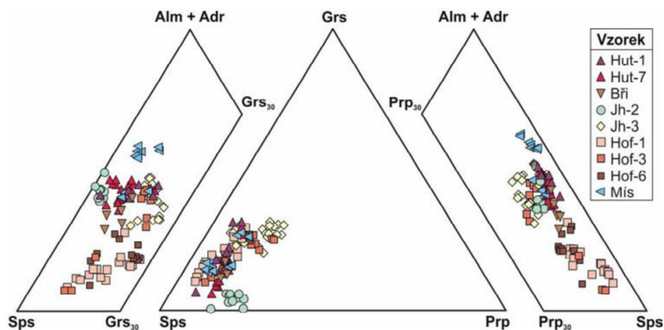
Obr. 53. Zastoupení jednotlivých komponent v granátech z granátovců a páskovaných železných rud z lokalit Hutisko, Jelení hřbet, Břidličná, Hofberg a Mísečky, vyjádřené v ternárních diagramech Sps–Alm+Adr–Grs 30 ; Sps–Grs–Prp; Sps–Alm+Adr–Prp 30 (Kropáč 2012).
