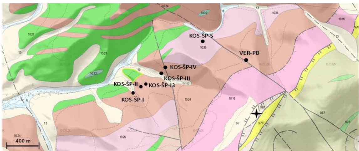
Obr. 12. Zaznačené navštívěné lokality v okolí Vernířovic. Vernířovice – Pod Břidličnou (VER-PB), Kosaře – Špičák – štola 5 (KOS-ŠP-5), Kosaře – Špičák – štola IV (KOS-ŠP-IV), Kosaře – Špičák – štola III (KOS-ŠP-III), Kosaře – Špičák – štola II (KOS-ŠP-II), Kosaře – Špičák – štola I (KOS-ŠP-I). Zdroj: Mapy.cz ( https://mapy.cz/turisticka?l=0&x=17.1667264&y=50.0359057&z=15 ).
