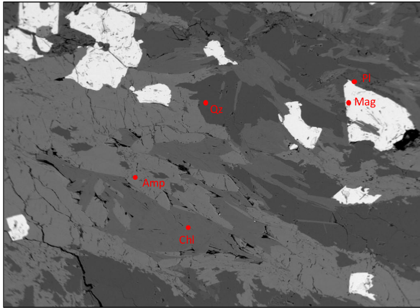
Obr. 33. Prorůstání chloritu a amfibolu, místy patrně dochází k zatlačování amfibolu chloritem. Vzorek KOS-ŠP-23. BSE snímek. Šířka snímku 1,5 mm. Foto: P. Gadas
