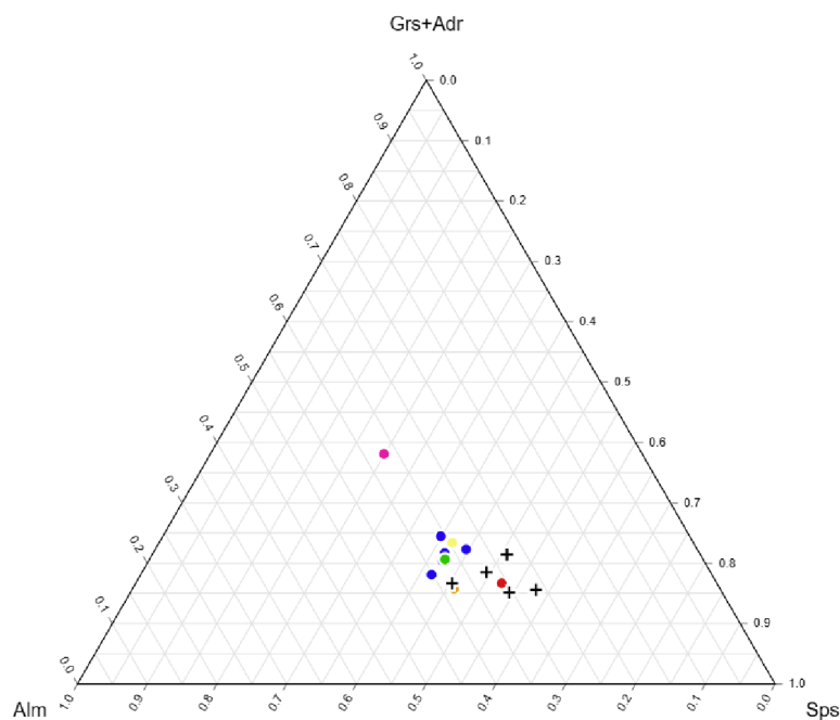
Obr. 47. Pozice granátů v systému Alm – Sps – Grs+Adr. Černé křížky zobrazují pozice analyzovaných granátů z lokality Pod Břidličnou. Barevná kolečka jsou analyzované granáty z lokality Kosaře-Špičák.
