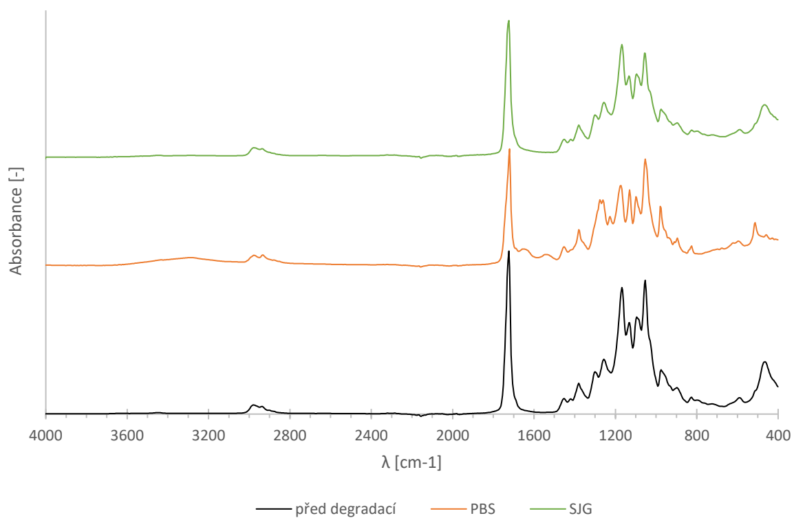
Obrázek P2: FTIR spektrum amorfního PHA – před degradací a po degradaci v PBS a SJG
