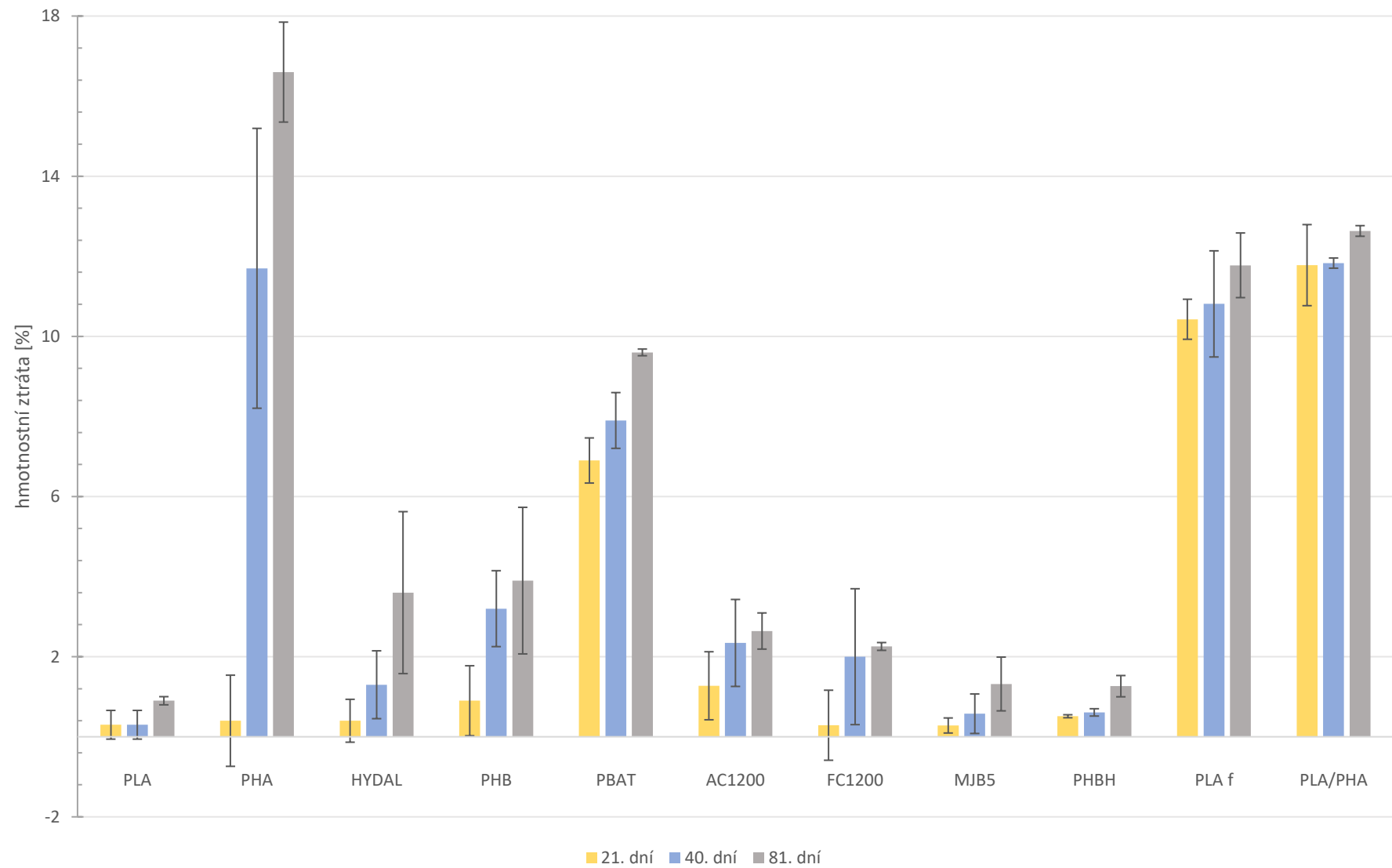
Obrázek 14: Hmotnostní úbytek v SGJ
