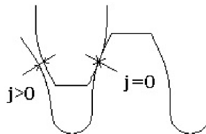
Obr. 3.14 Boční vůle
