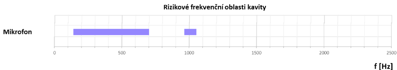
Obr. 8.45 Rizikové frekvenční oblasti pramenící z rezonančních vlastností kavity
