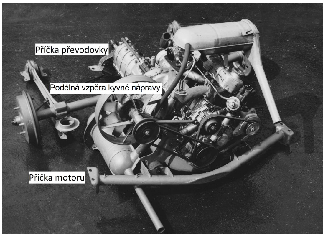
Obr. 4.3 Uložení agregátu Škoda 1000MB či Škoda 742
