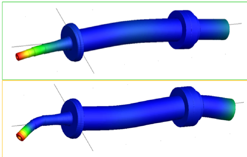
Obr. 7.2 Tabulka některých vypočtených vlastních frekvencí primárního hřídele stavu na chybu převodu a některé vlastní tvary kmitu
