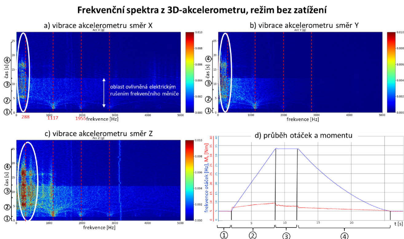
Obr. 8.34 Rozběhová a doběhová zkouška PST-TE s přímým zapojením bez zatížení (tj. při pasivních odporech Haldexu) a)b)c) - Záznam z 3D akcelerometru (směry x, y, z) d) modrá – frekvence otáček elektromotoru [Hz], červená – průměrovaný signál momentového snímače [Nm]
