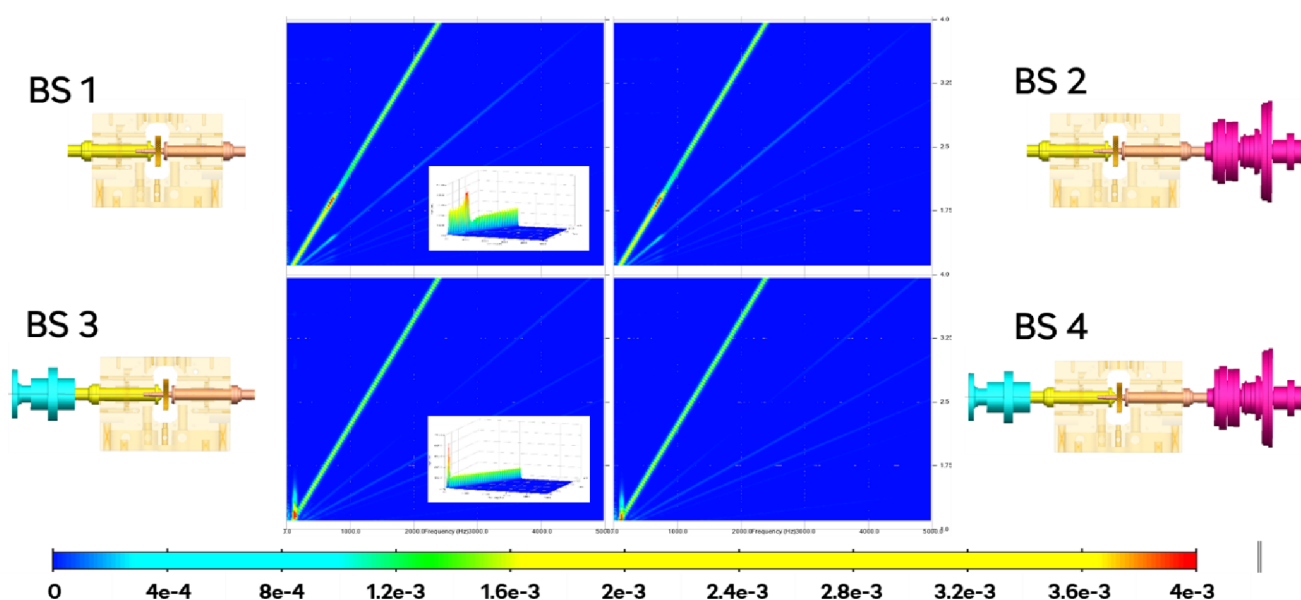
Obr. 7.10 Vliv rozsahu MBS modelu a jeho rotačních setrvačných hmot na výpočet TE
