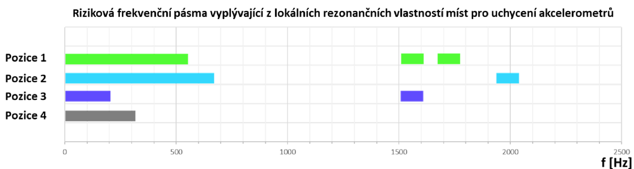
Obr. 8.31 Graf s vyznačenými rizikovými frekvenčními pásmy v pozicích umístění akcelerometrů
