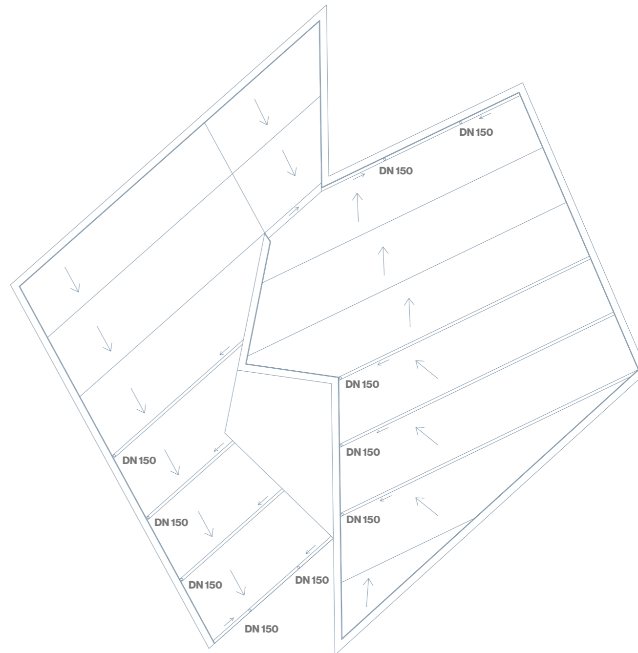
schéma vyřešení odtoku vody
