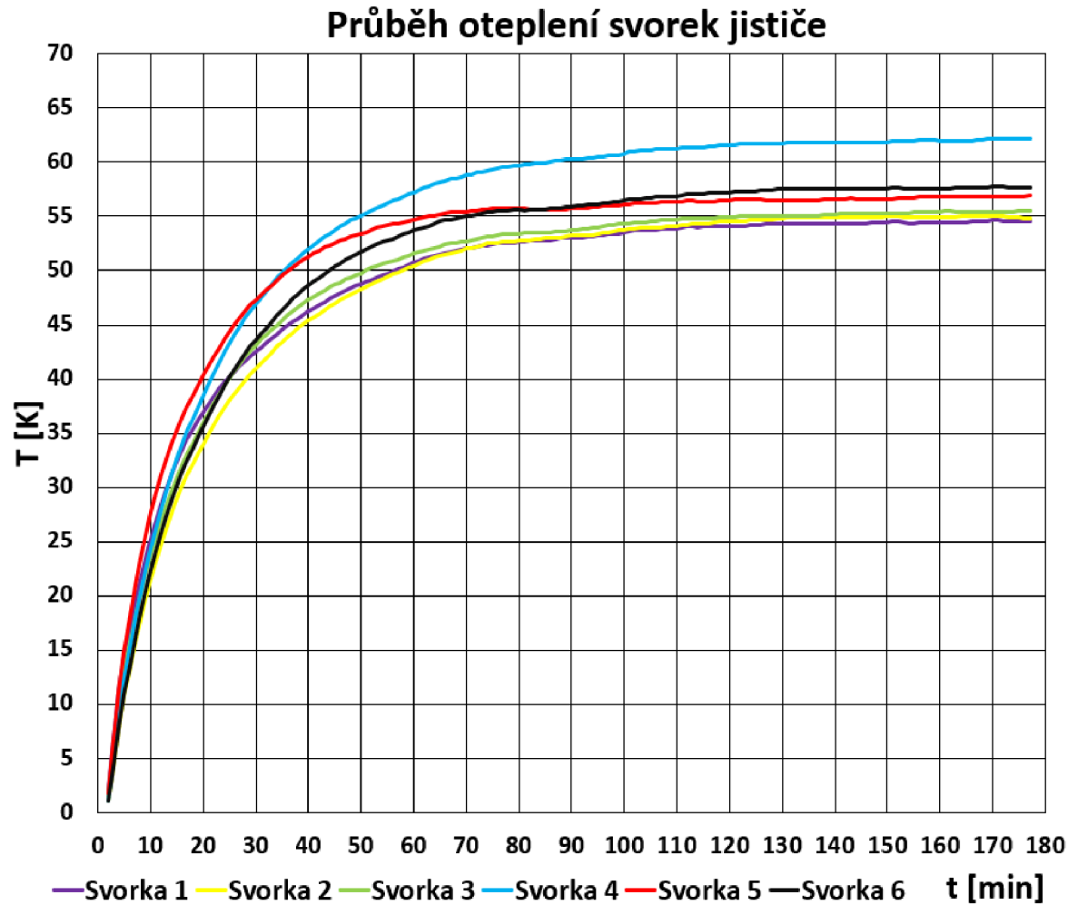
Obr. 7.2: Graf průběhu oteplení jednotlivých svorek jističe
