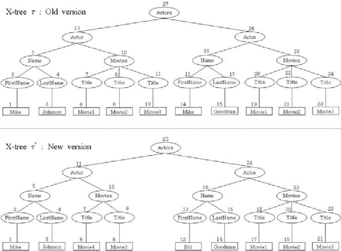
Obrázek 2.4: Příklad X-tree[17]
