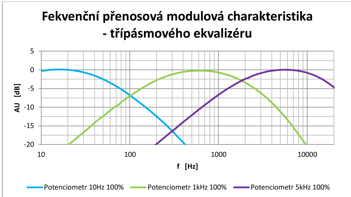
Obr. 45 Frekvenční přenosová modulová charakteristika třípásmového ekvalizéru (jednotlivá pásma)
