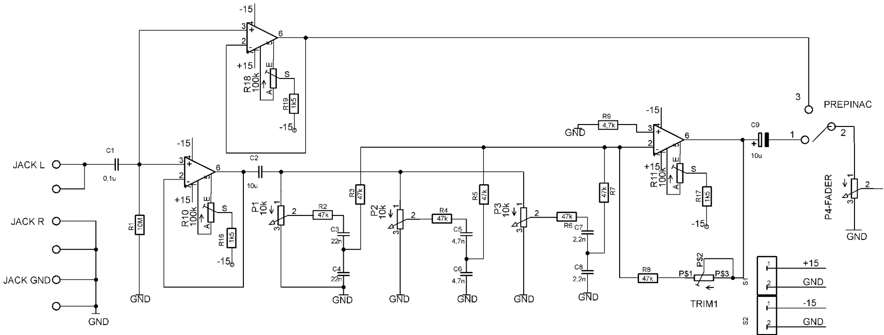
Obr. 13: Schéma zapojení třípásmového ekvalizéru
