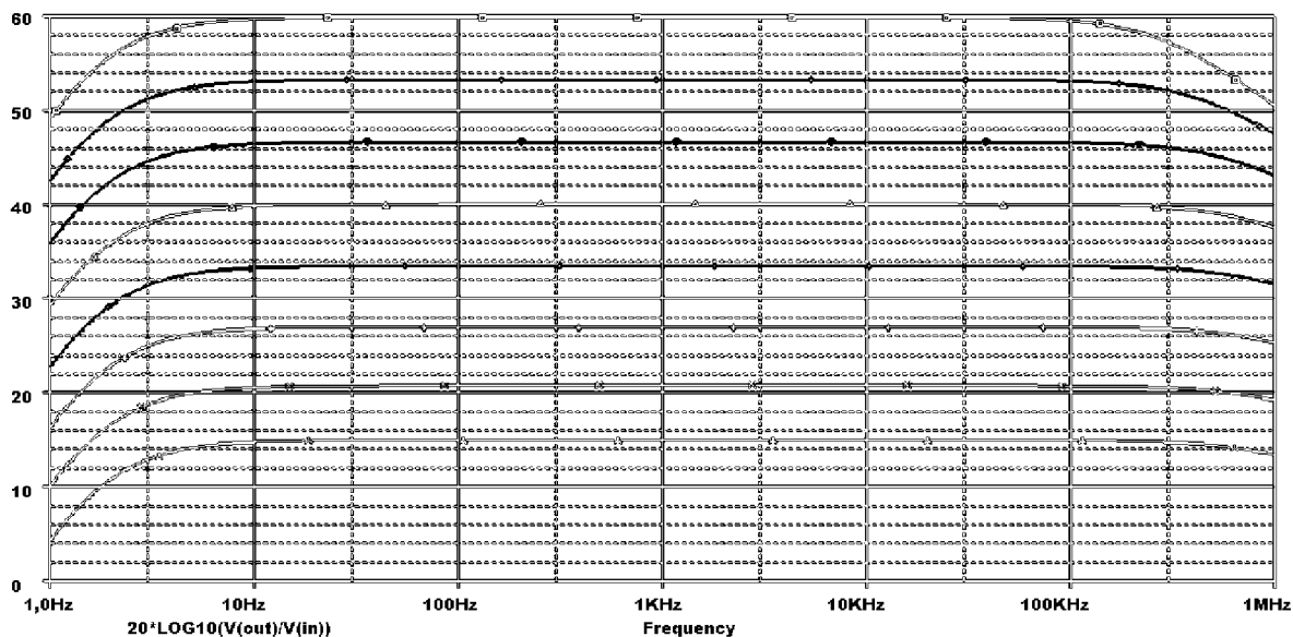
Obr. 6: Průběh frekvenční přenosové modulové charakteristiky mikrofonního předzesilovače při rozmitání hodnoty odporu R_G
