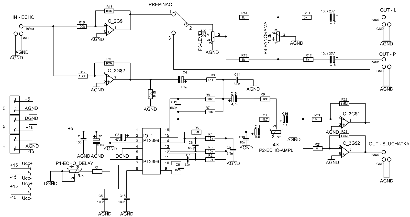
Obr. 12: Obvodové schéma zapojení echo processoru PT2399.
