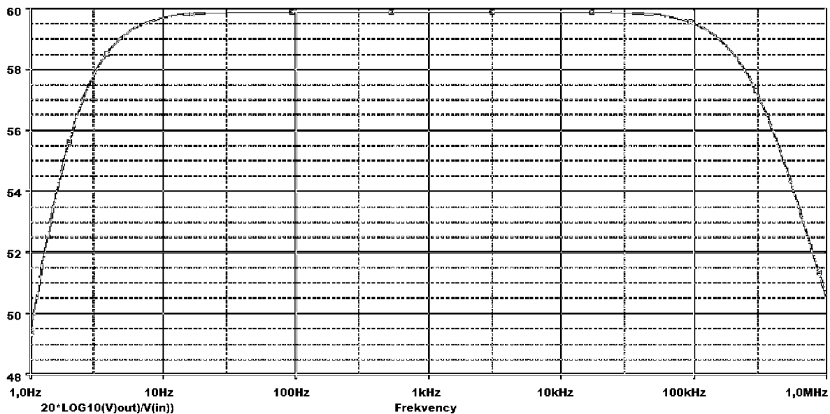
Obr. 5: Průběh frekvenční přenosové modulové charakteristiky mikrofonního předzesilovače
