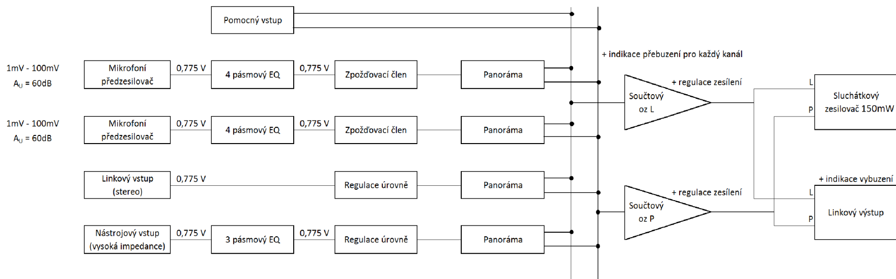
Obr. 2: blokové schéma zapojení mixážního pultu
