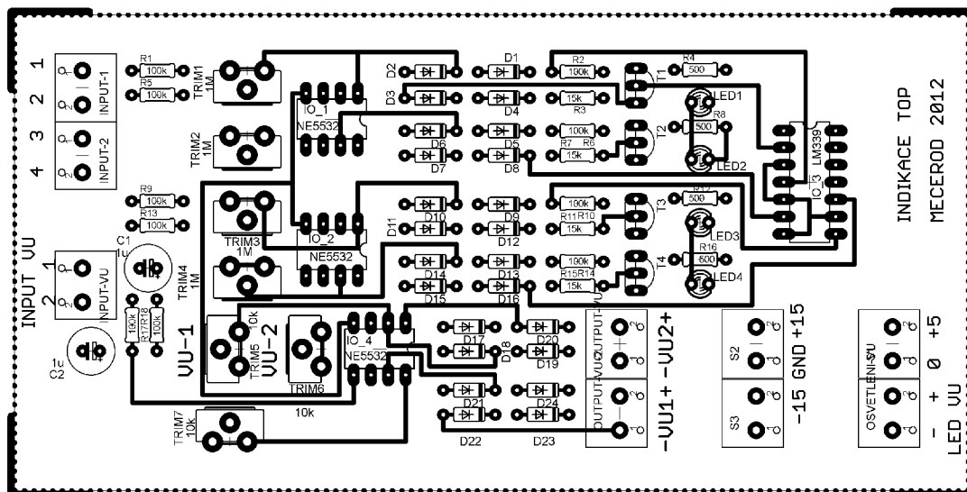
Obr. 41 Osazovací plán indikátorů (140x70)mm, M1:1 Seznam součástek Tab.29
