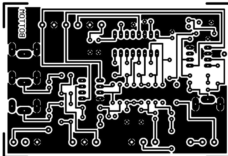
Obr. 28 DPS zpožďovacího členu (BOTTOM) (95x64)mm, M1:1
