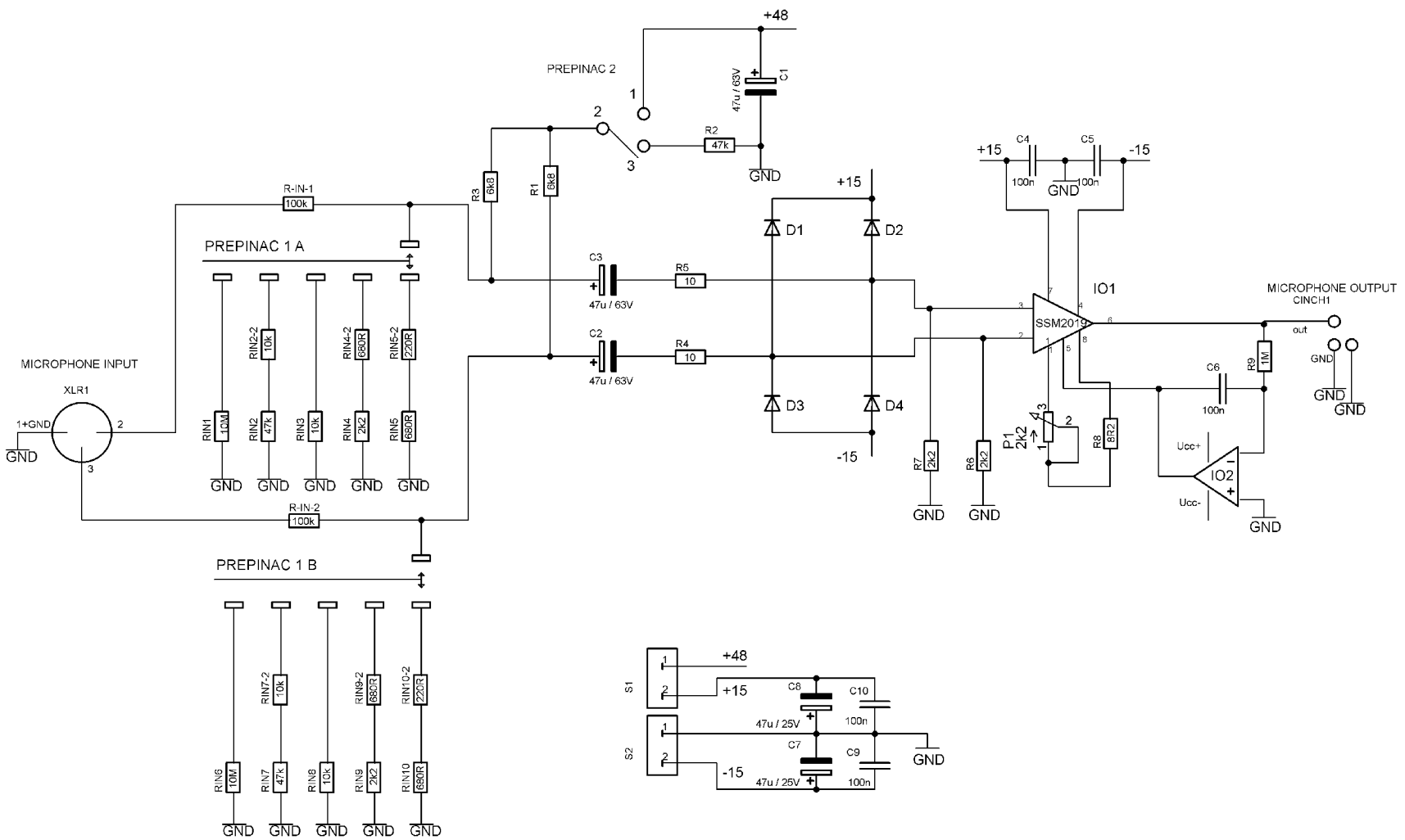
Obr. 4: Schéma zapojení mikrofonního předzesilovače
