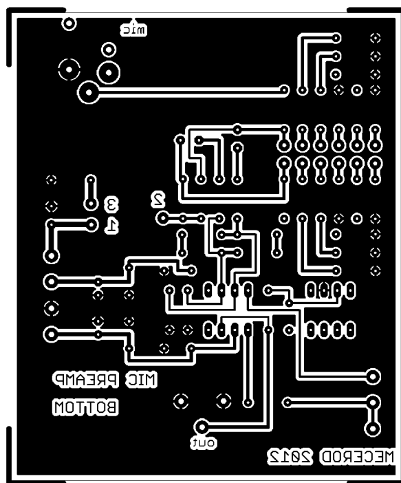
Obr. 22 DPS mikrofonního předzesilovače (BOTTOM) (75x90)mm, M1:1
