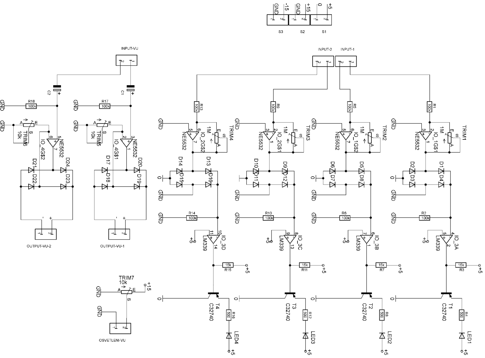
Obr. 20 Schéma zapojení indikátorů
