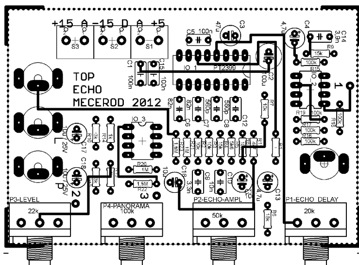
Obr. 29 Osazovací plán zpožďovacího členu (95x64)mm, M1:1 Seznam součástek Tab.25
