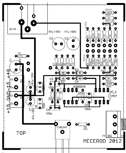
Obr. 23 Osazovací plán mikrofonního předzesilovače (75x90)mm, M1:1 Seznam součástek Tab.23
