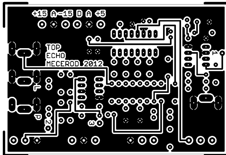
Obr. 27 DPS zpožďovacího členu (TOP) (95x64)mm, M1:1
