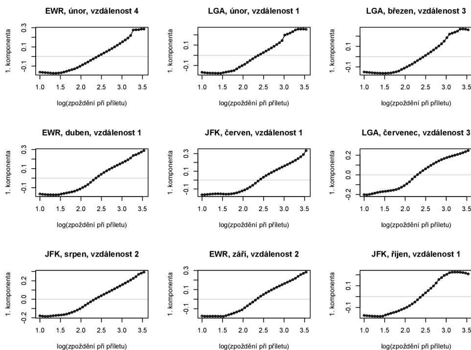
Obrázek 14: První komponenty singulárních rozkladů interakčních částí hustot odpovídající zlogaritmovanému zpoždění při přeletu.
